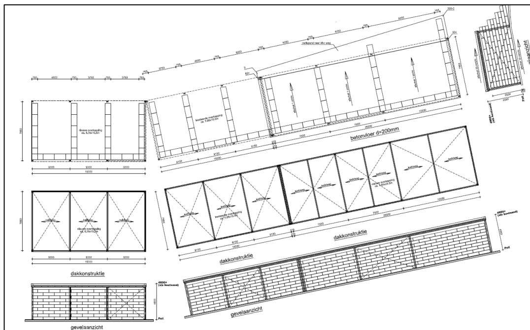
Uitbreiding overkapping
