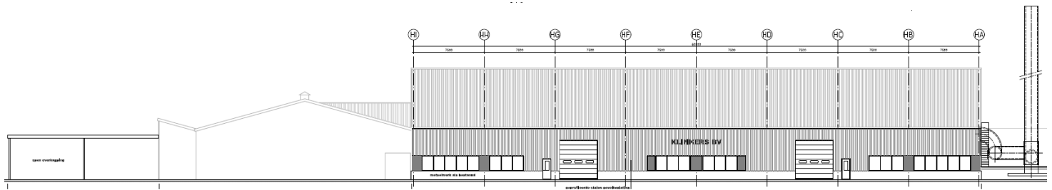
Aanzicht westgevel
