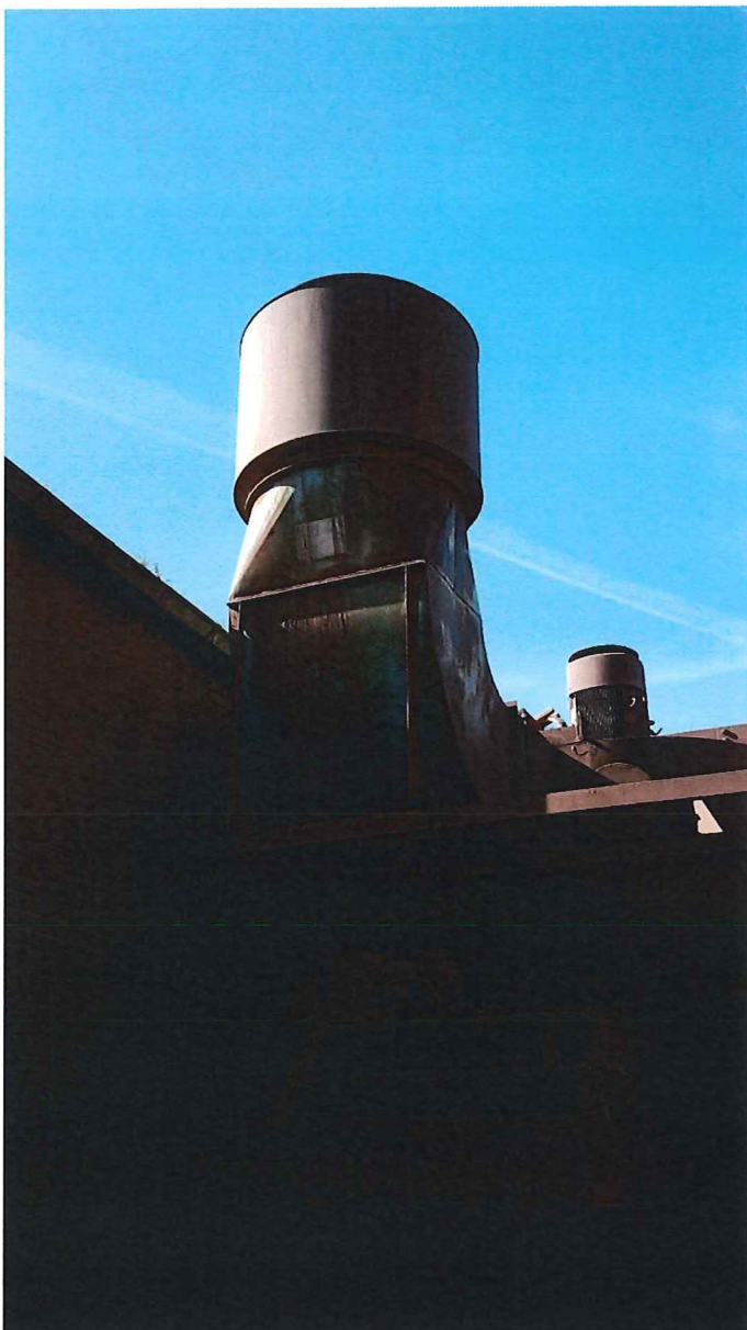
Foto 1: Afgasleiding natwasser na de ventilator.
