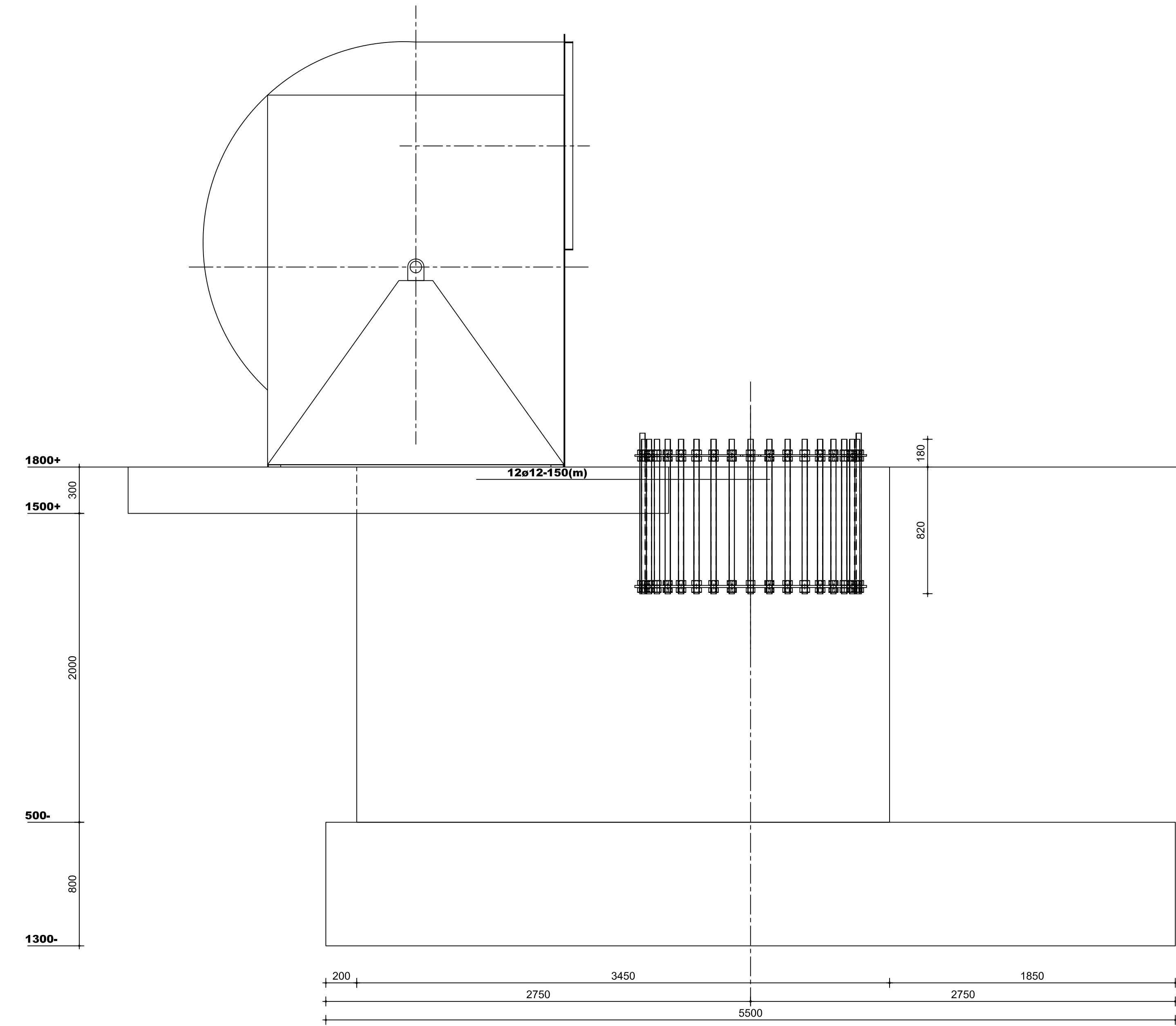
Fundering schoorsteen zijaanzicht
