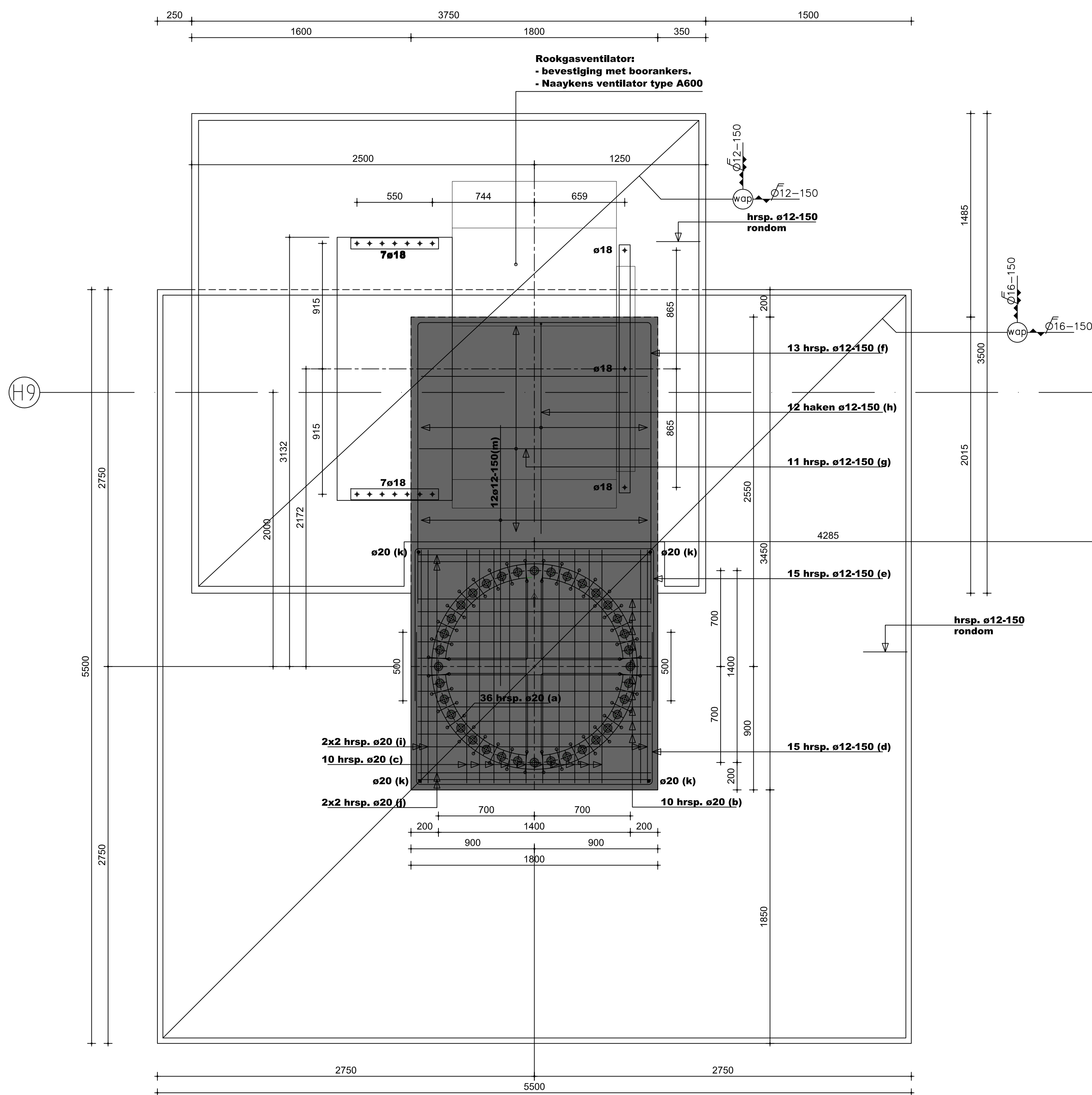
Fundering schoorsteen bovenaanzicht
