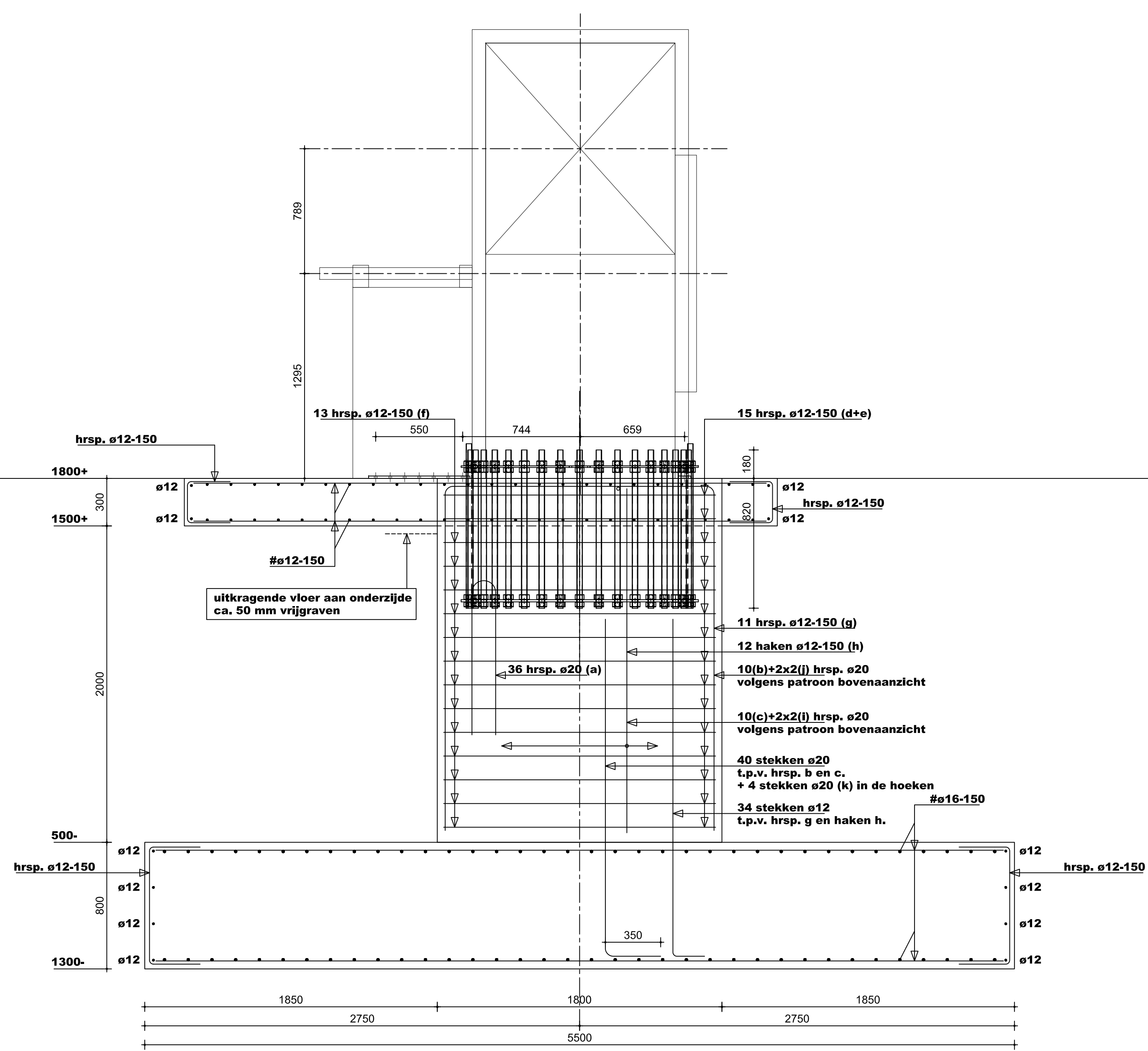
Fundering schoorsteen vooraanzicht
