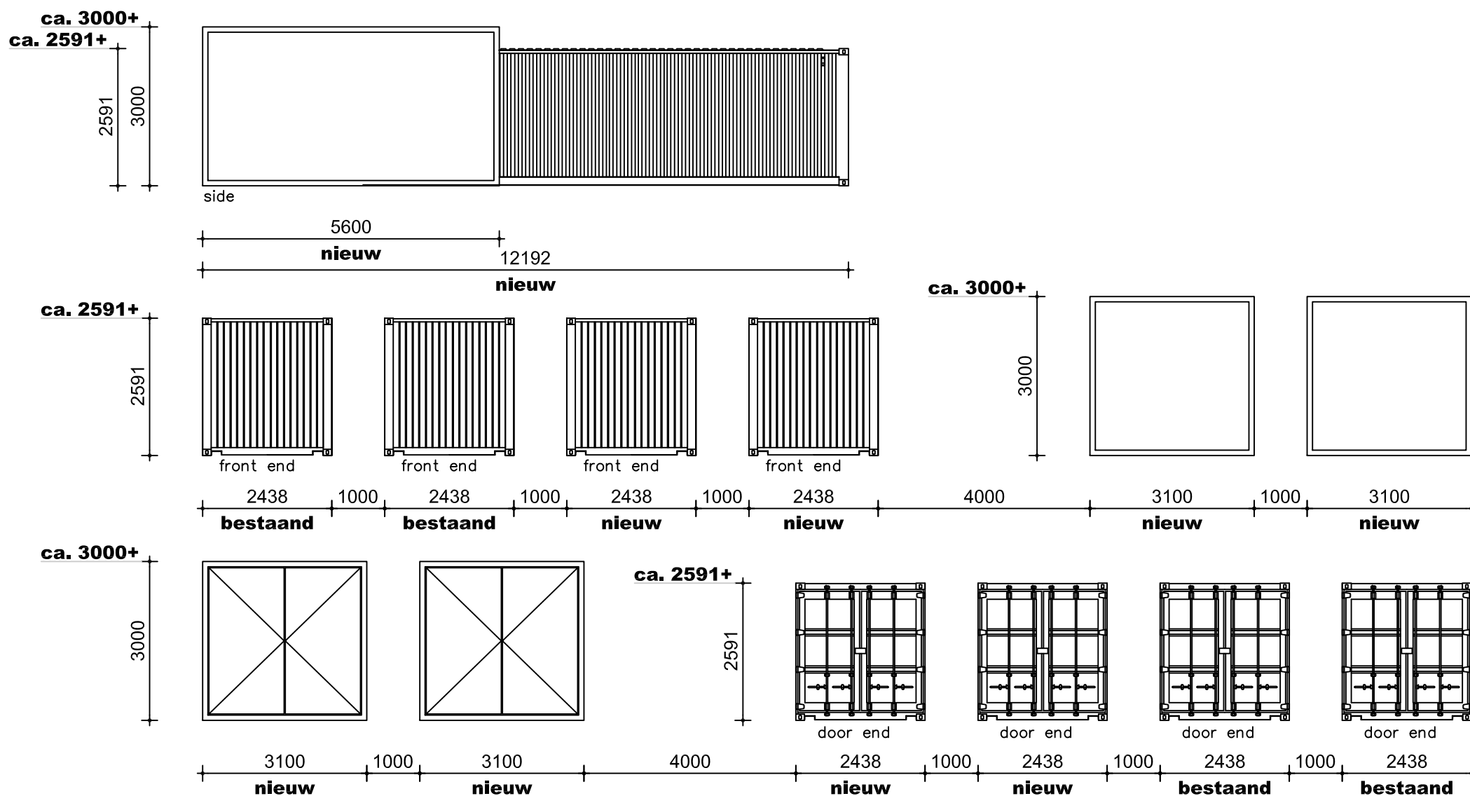
aanziichten containers
