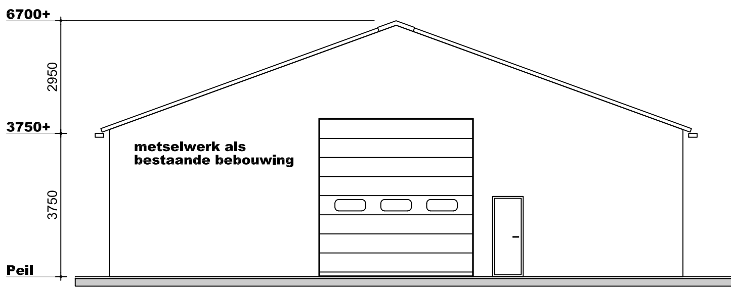
Oostgevel
