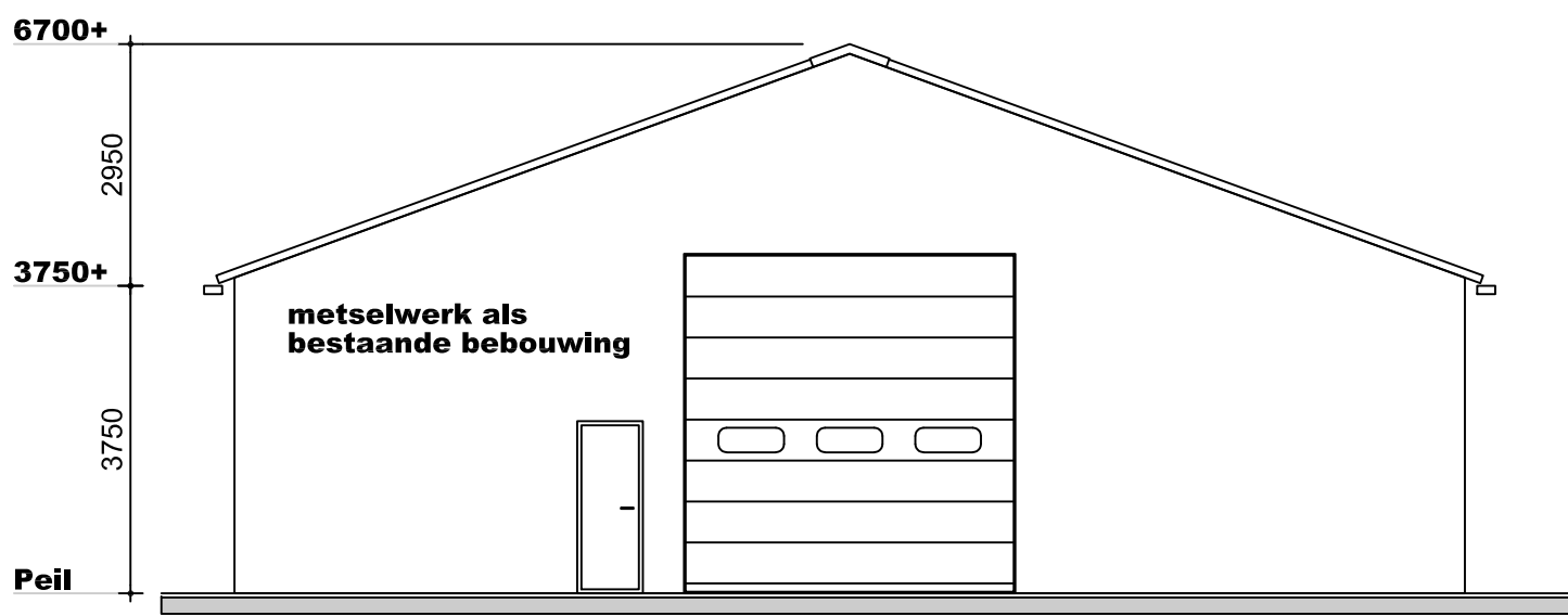
Westgevel
