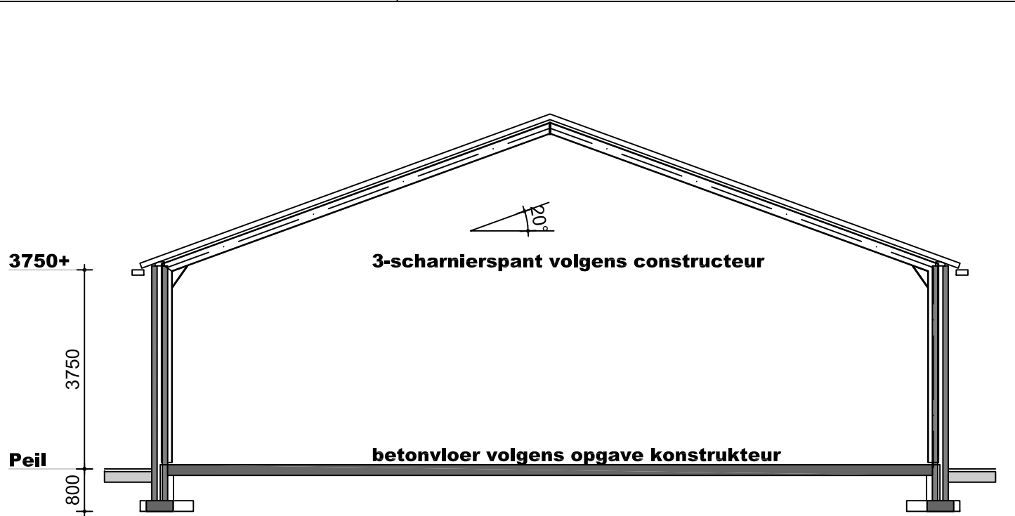
Doorsnede B-B
