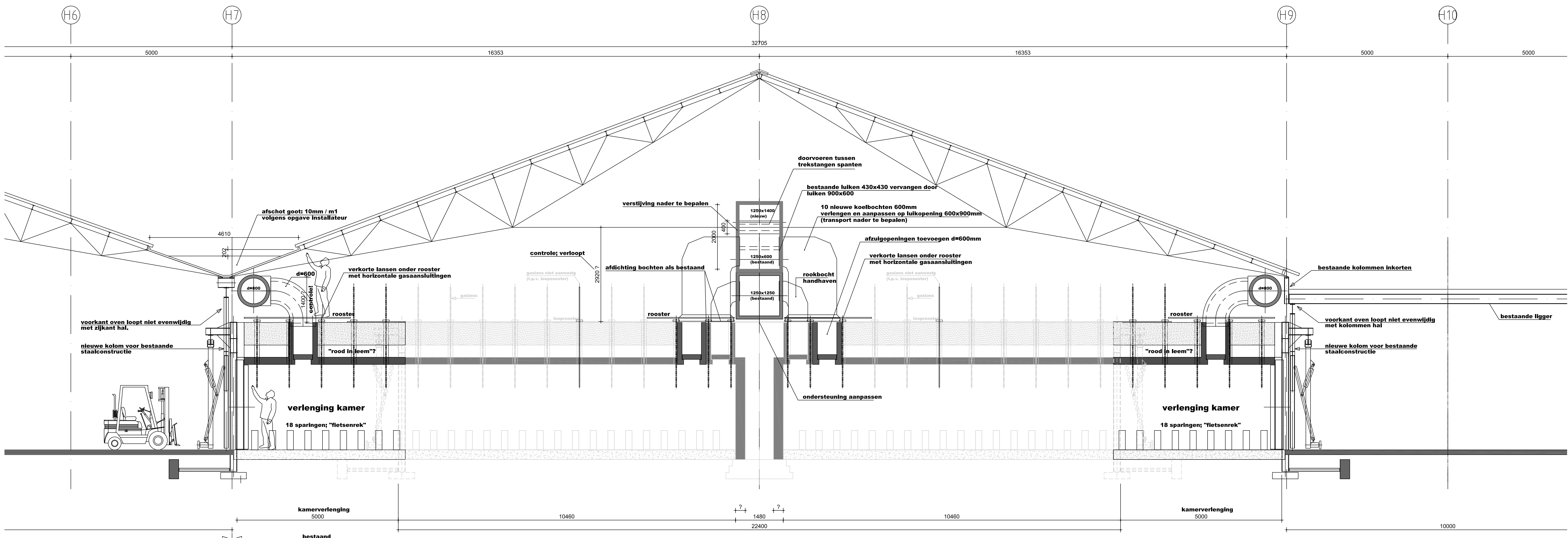
Doorsnede A-A NIEUWE SITUATIE
