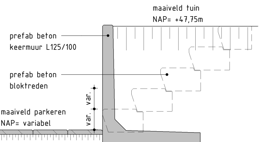
Detail keermuur beton
