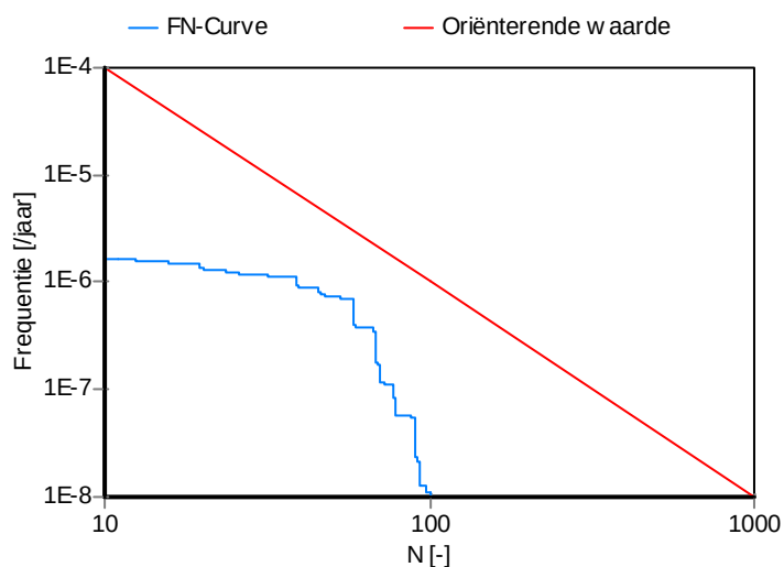
Figuur 5 FN-curve Z-500-15-KR-001 t/m 010 voor scenario 5. Overschrijdingsfactor 0.23
