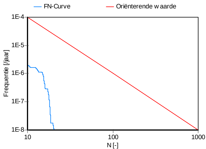
Figuur 3 FN-curve Z-500-15-KR-001 t/m 010 voor scenario 3. Overschrijdingsfactor 0.02
