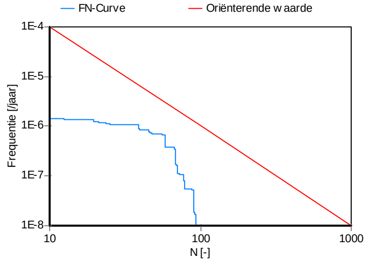
Figuur 2 FN-curve Z-500-15-KR-001 t/m 010 voor scenario 2. Overschrijdingsfactor 0.23
