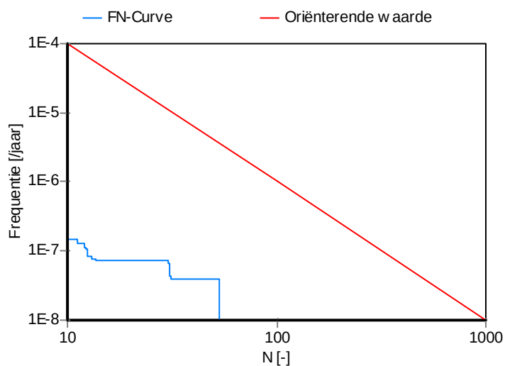
Figuur 4 FN-curve Z-500-15-KR-001 t/m 010 voor scenario 4. Overschrijdingsfactor 0.01
