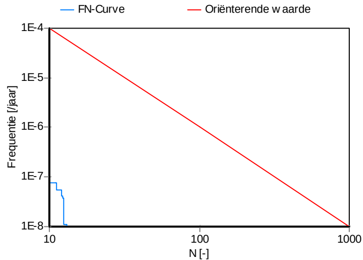
Figuur 1 FN-curve Z-500-15-KR-001 t/m 010 voor scenario 1. Overschrijdingsfactor 0.00
