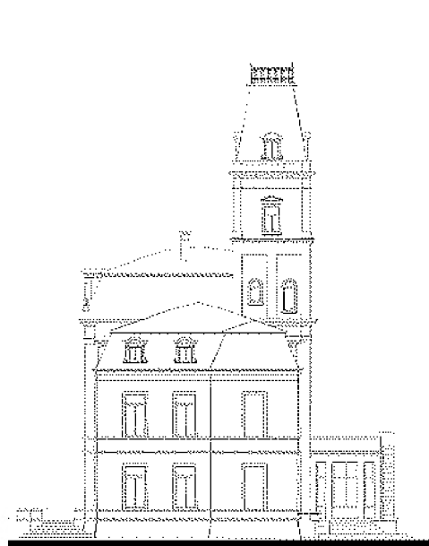
rechter zijgevel Villa Kanjel
