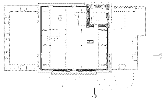
3e verdieping Villa Kanjel
