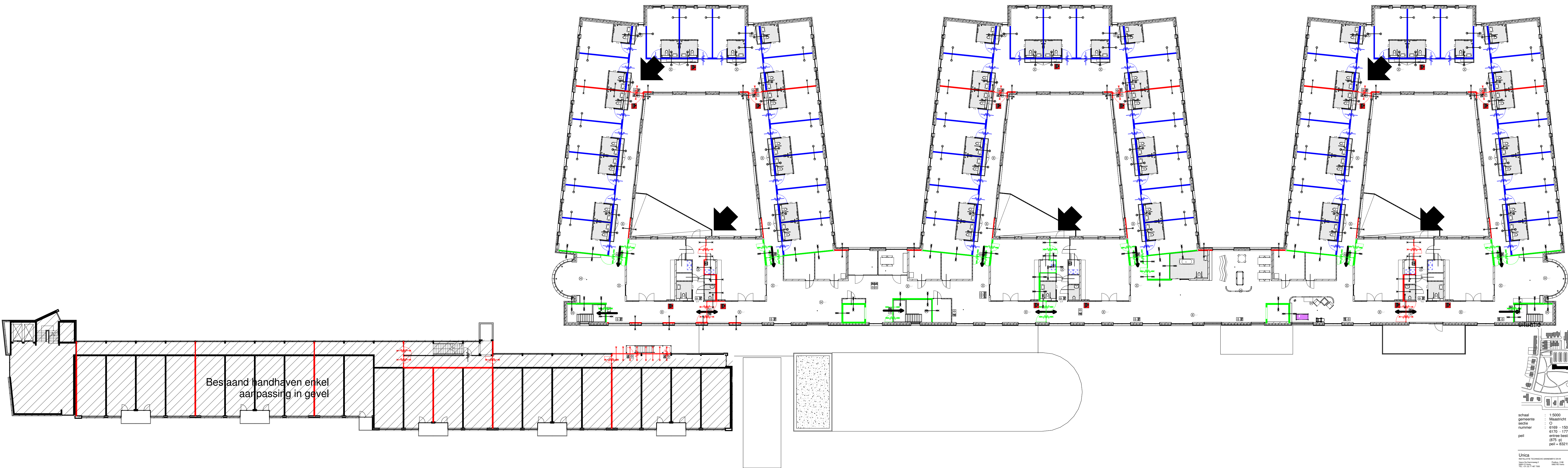
Brandscheiding 2e verdieping
