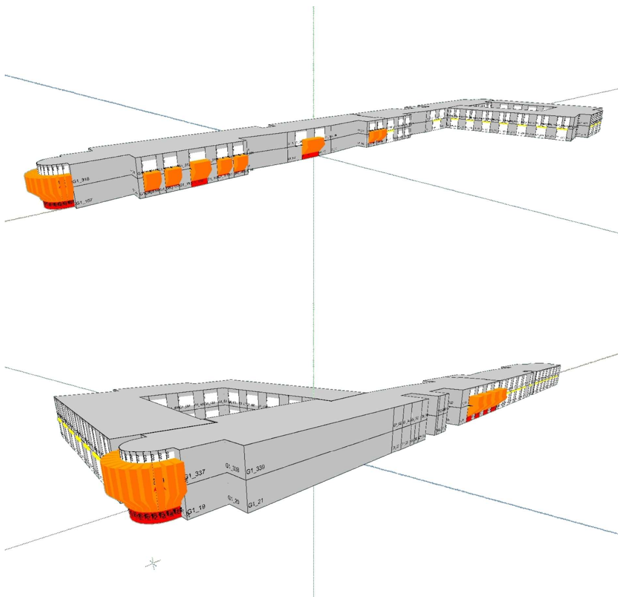
Figuur 3: voorgevel + achtergevel in brandsituatie
