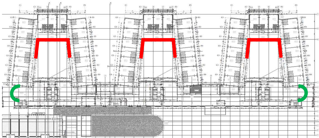
Figuur 5: locaties brandwerende beglazing vereist (rood + groen aangestreepte gevelopeningen)
