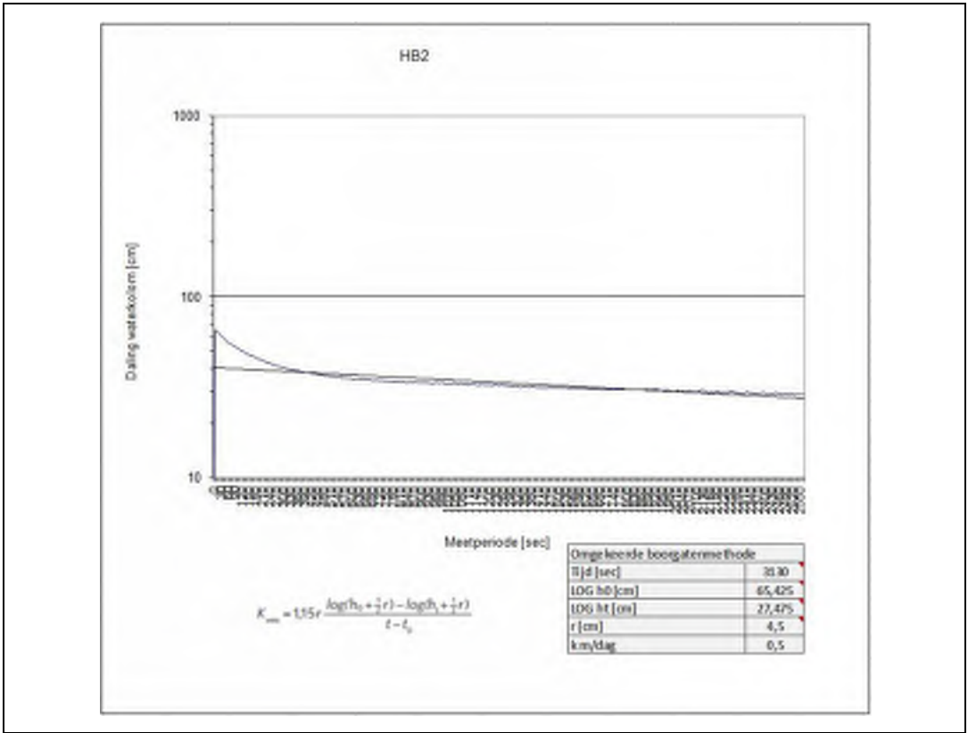
Infiltratiemeting HB2.
