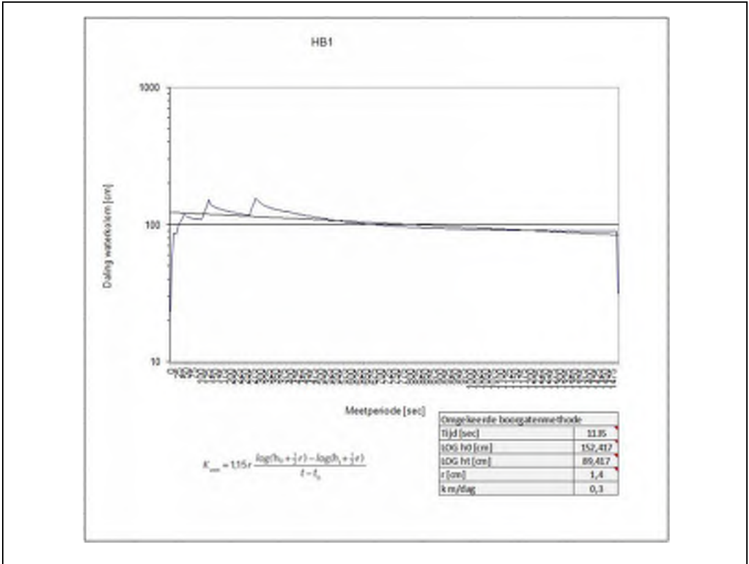
Infiltratiemeting HB1.
