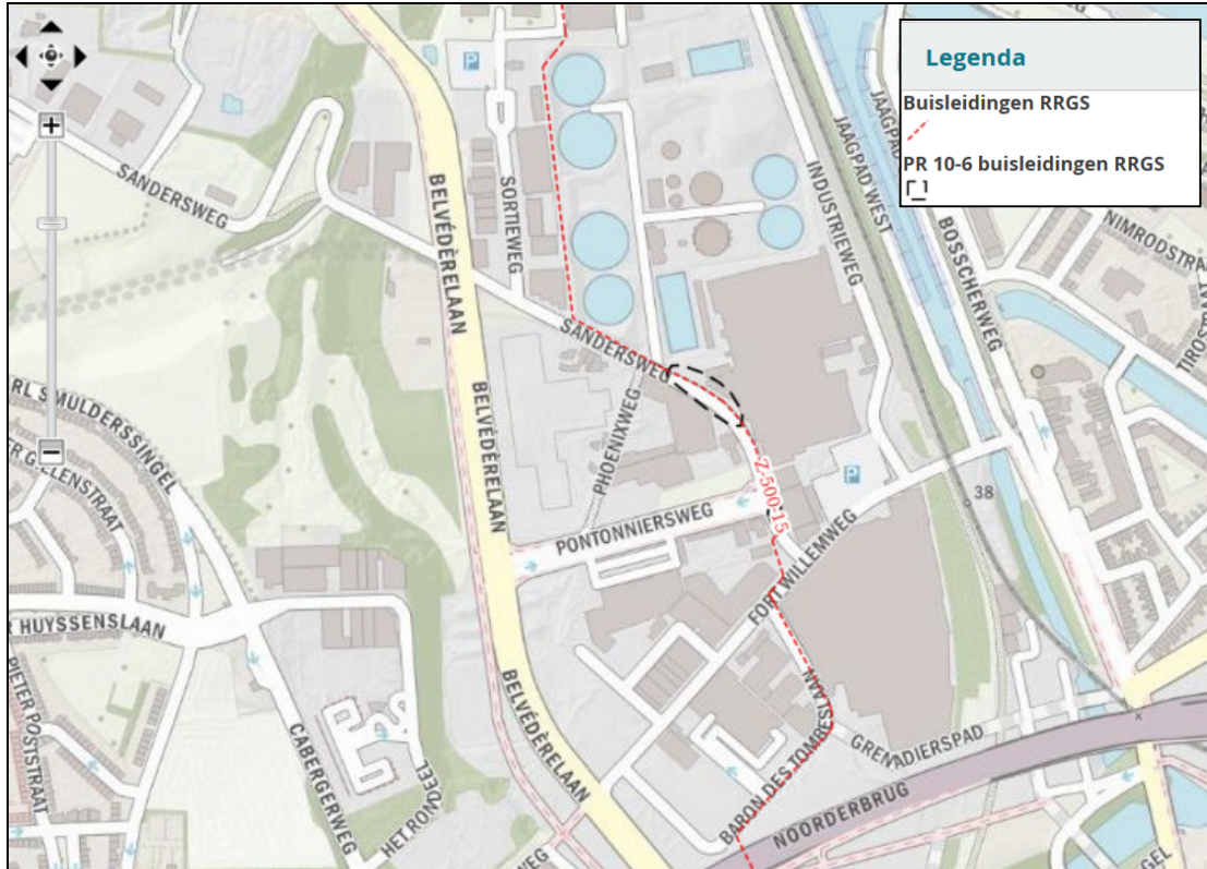
Figuur 1: Ligging hoge druk aardgasleiding en PR 10 -6 - contour
