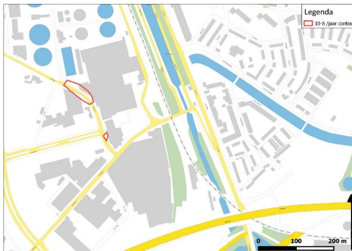
Figuur 6.1: PR 10^{-6} -contouren hogedruk aardgastransportleiding
