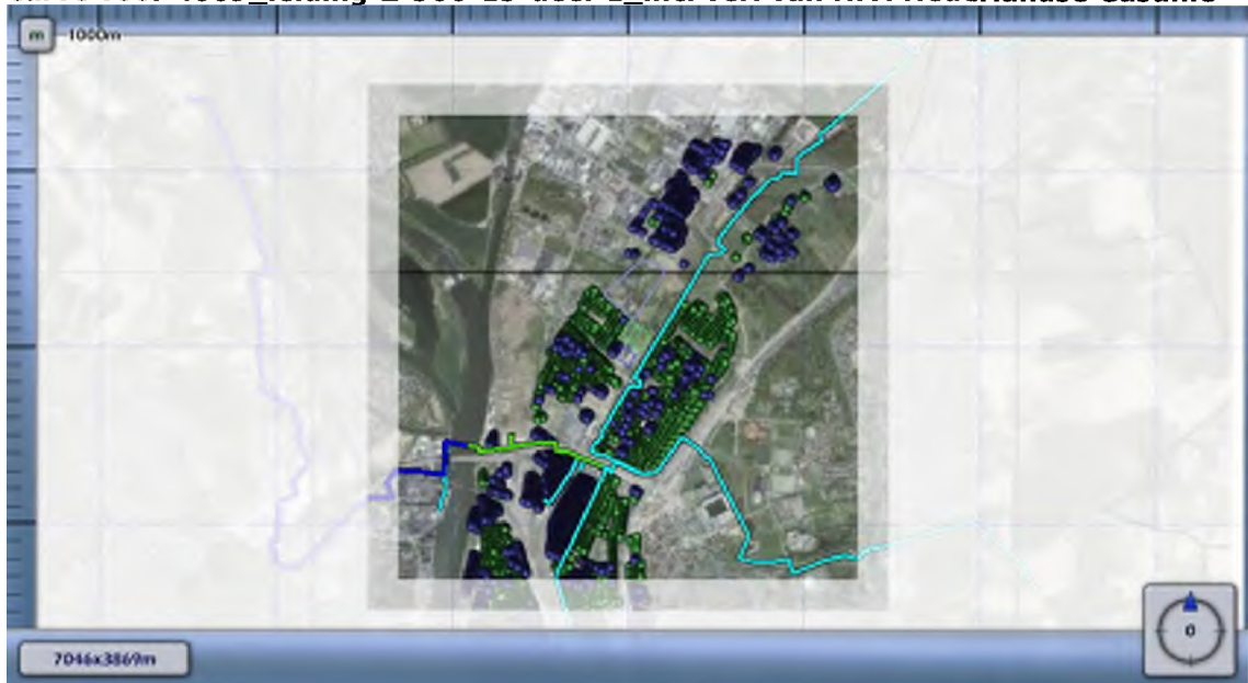
Figuur 4.13 Kilometer leiding behorende bij de maximale overschrijding van de FN-curve voor 4609 leiding-Z-500-15-deel-1_incl verl van N.V. Nederlandse Gasunie
