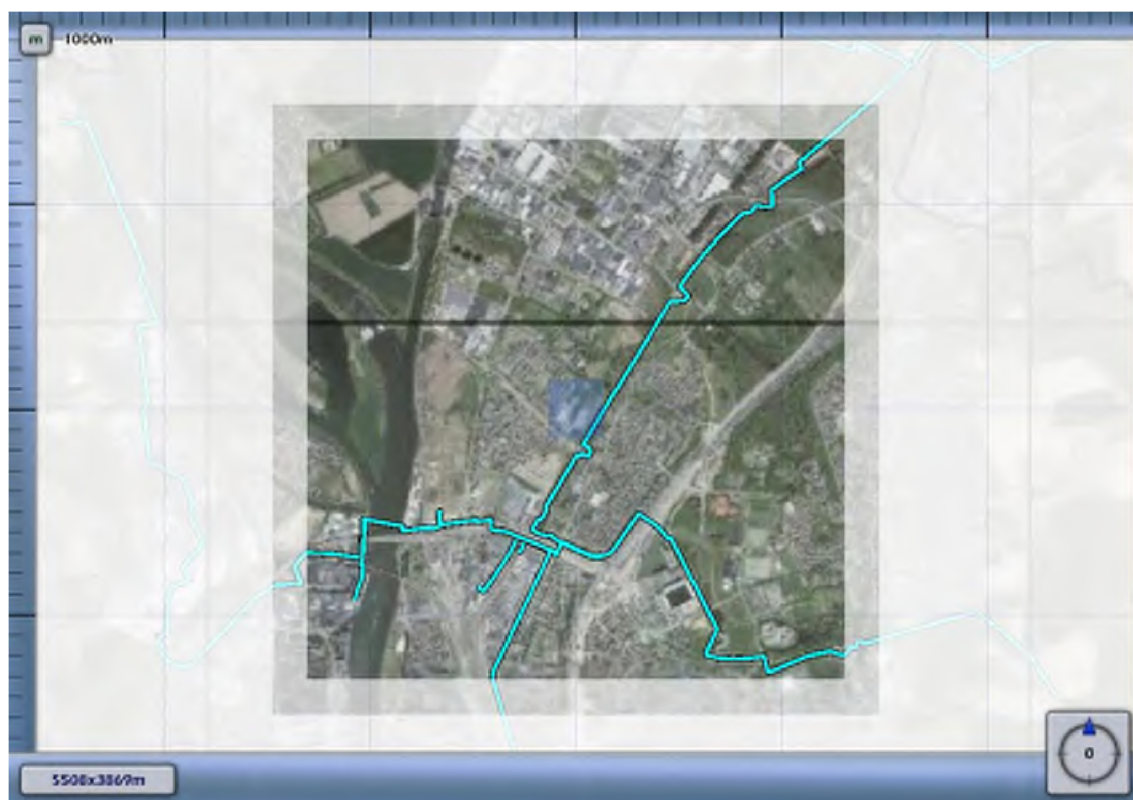
3.10 Figuur 3.10 Plaatsgebonden risico voor 4608_leiding-Z-530-01-deel-1 van N.V. Nederlandse Gasunie
