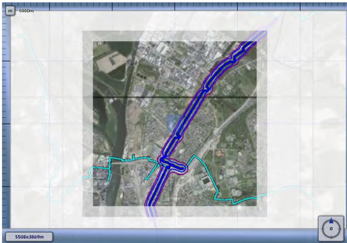
3.1 Figuur 3.1 Plaatsgebonden risico voor 4608_leiding-Z-500-01-deel-1 van N.V. Nederlandse Gasunie
