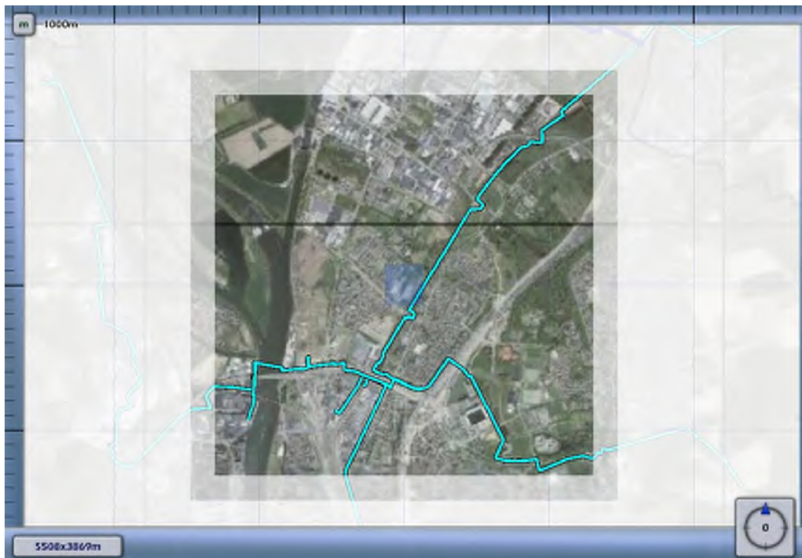
3.12 Figuur 3.12 Plaatsgebonden risico voor 4608_leiding-Z-530-17-deel-1 van N.V. Nederlandse Gasunie
