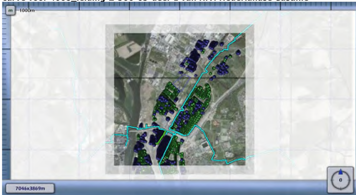
Figuur 4.3 Kilometer leiding behorende bij de maximale overschrijding van de FN-curve voor 4608_leiding-Z-500-05-deel-1 van N.V. Nederlandse Gasunie
