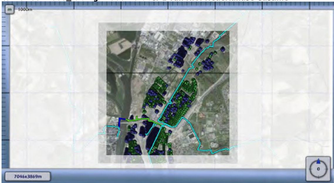
Figuur 4.7 Kilometer leiding behorende bij de maximale overschrijding van de FN-curve voor 4608_leiding-Z-500-16-deel-1 van N.V. Nederlandse Gasunie
