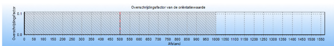
4.13 Figuur 4.13 Groepsrisico screening voor 4609_leiding-Z-500-15-deel-1_incl verl van N.V. Nederlandse Gasunie
