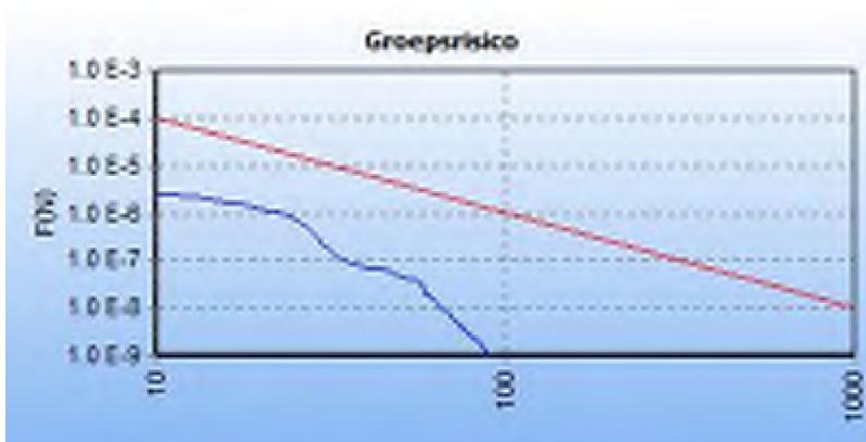
5.2 Figuur 5.2 FN curve voor 4608_leiding-Z-500-02-deel-1 van N.V. Nederlandse Gasunie voor de kilometer tussen stationing 0.00 en stationing 0.00
