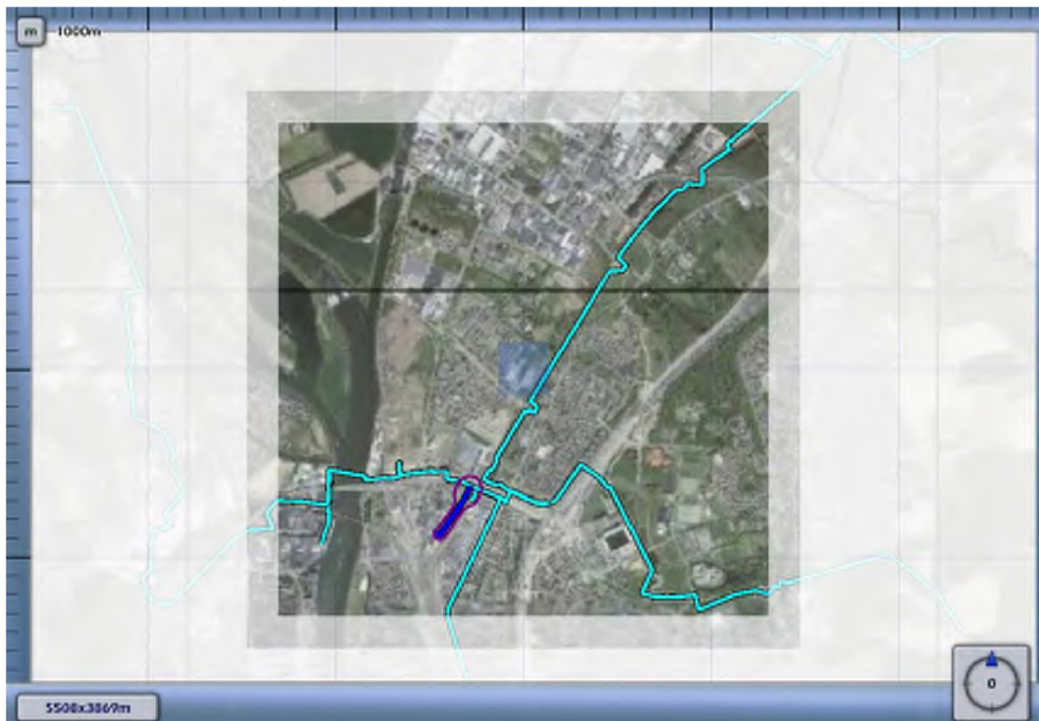
3.3 Figuur 3.3 Plaatsgebonden risico voor 4608_leiding-Z-500-05-deel-1 van N.V. Nederlandse Gasunie
