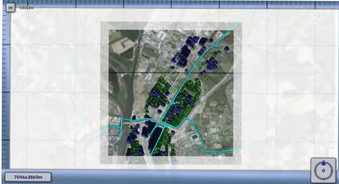
Figuur 4.10 Kilometer leiding behorende bij de maximale overschrijding van de FN-curve voor 4608_leiding-Z-530-01-deel-1 van N.V. Nederlandse Gasunie
