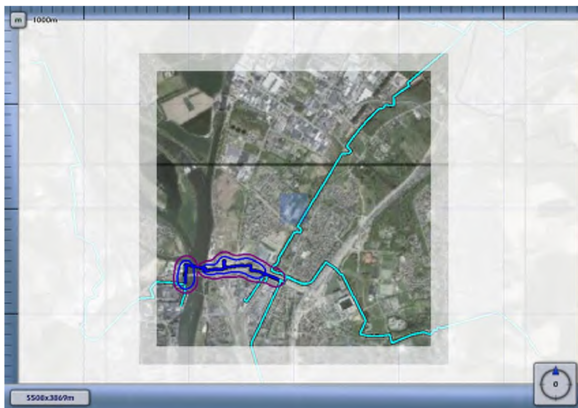
3.7 Figuur 3.7 Plaatsgebonden risico voor 4608_leiding-Z-500-16-deel-1 van N.V. Nederlandse Gasunie
