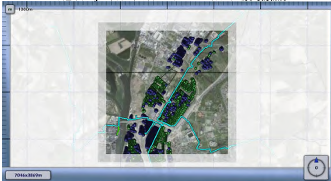
Figuur 4.8 Kilometer leiding behorende bij de maximale overschrijding van de FN-curve voor 4608_leiding-Z-500-19-deel-1 van N.V. Nederlandse Gasunie
