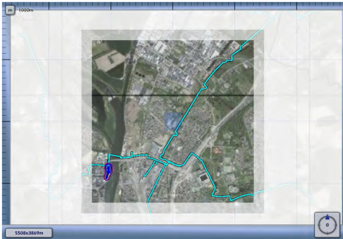
3.9 Figuur 3.9 Plaatsgebonden risico voor 4608_leiding-Z-501-01-deel-1 van N.V. Nederlandse Gasunie
