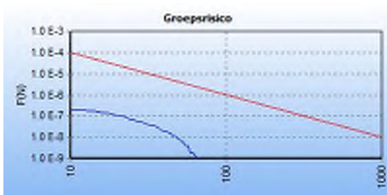
5.8 Figuur 5.8 FN curve voor 4608_leiding-Z-500-19-deel-1 van N.V. Nederlandse Gasunie voor de kilometer tussen stationing 0.00 en stationing 230.00
