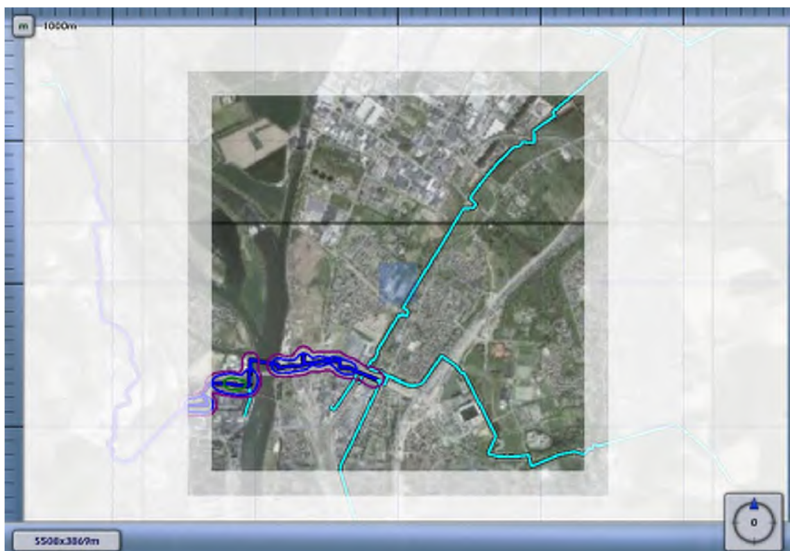
3.6 Figuur 3.6 Plaatsgebonden risico voor 4608_leiding-Z-500-15-deel-1_excl verl van N.V. Nederlandse Gasunie
