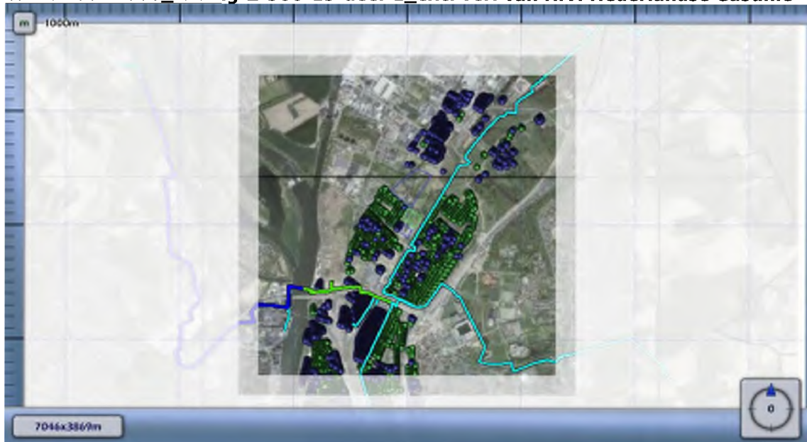
Figuur 4.6 Kilometer leiding behorende bij de maximale overschrijding van de FN-curve voor 4608_leiding-Z-500-15-deel-1_excl verl van N.V. Nederlandse Gasunie
