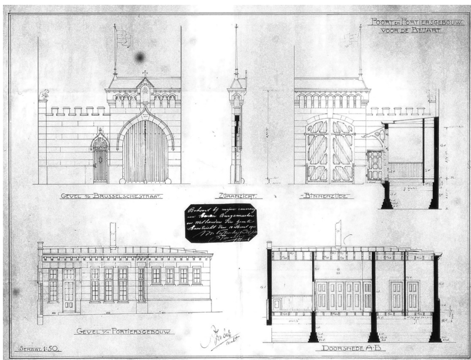
40 ontwerptekening voor het poortgebouw door Faber, gevelaanzichten en doorsneden.
