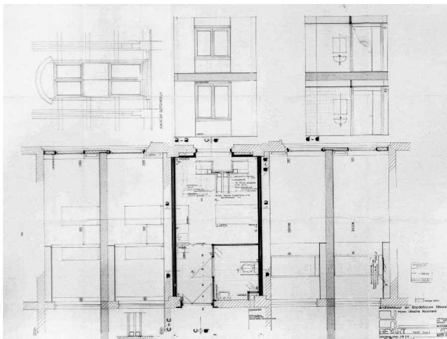
37 Bouwtekening 1981. Principedetail standaard wooneenheid in de tussenverdieping van de hoofdbouw..
