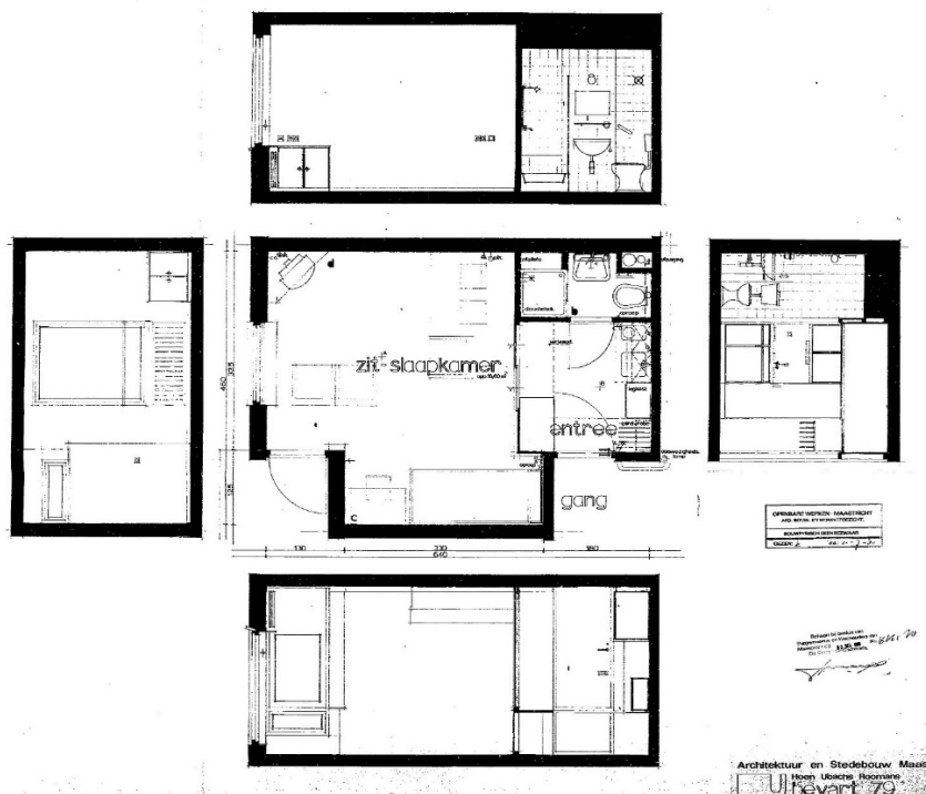
34 Bouwtekening 1980. Footprint standaard wooneenheid in de nieuwe woonvleugel.
