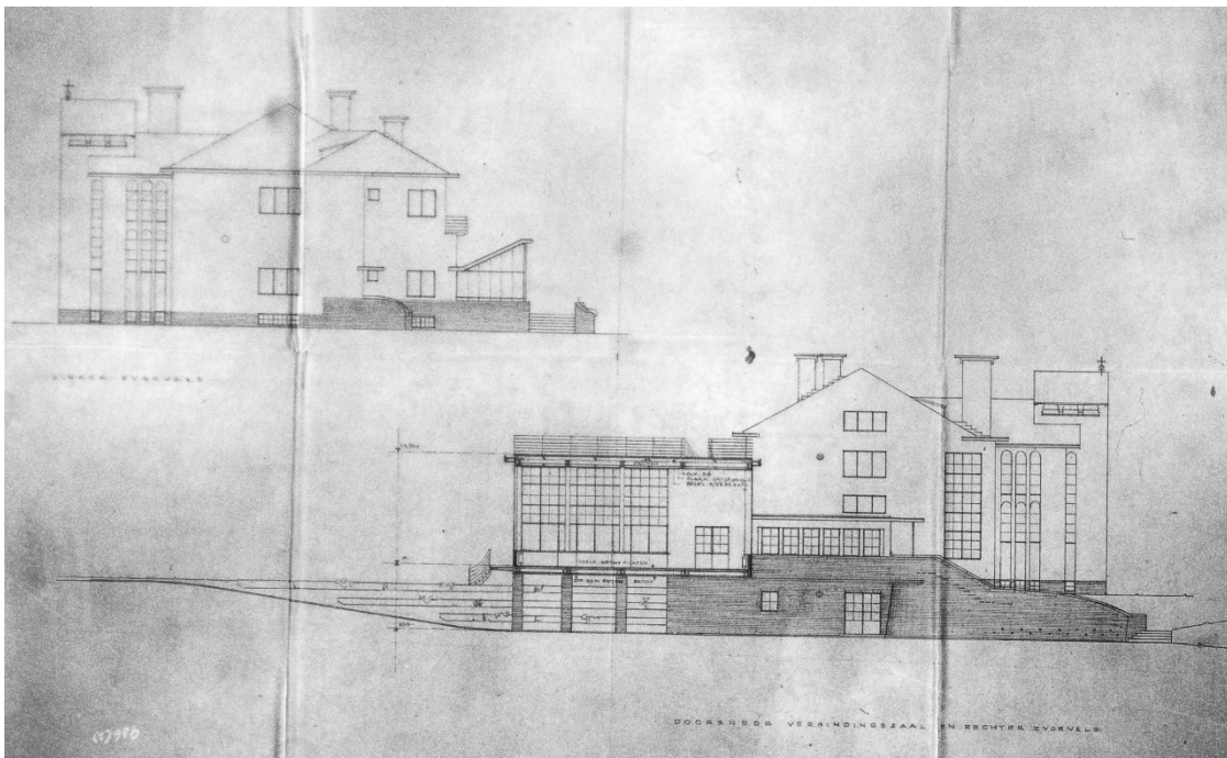
47 Ontwerptekening voor het Lydwina paviljoen: zijaanzielen kopgevels en doorsnede verbindingszaal.
