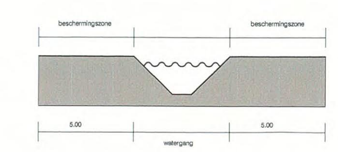
profiel (gerioleerde) watergang maten in meters
