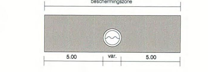
profiel (gerioleerde) watergang maten in meters
