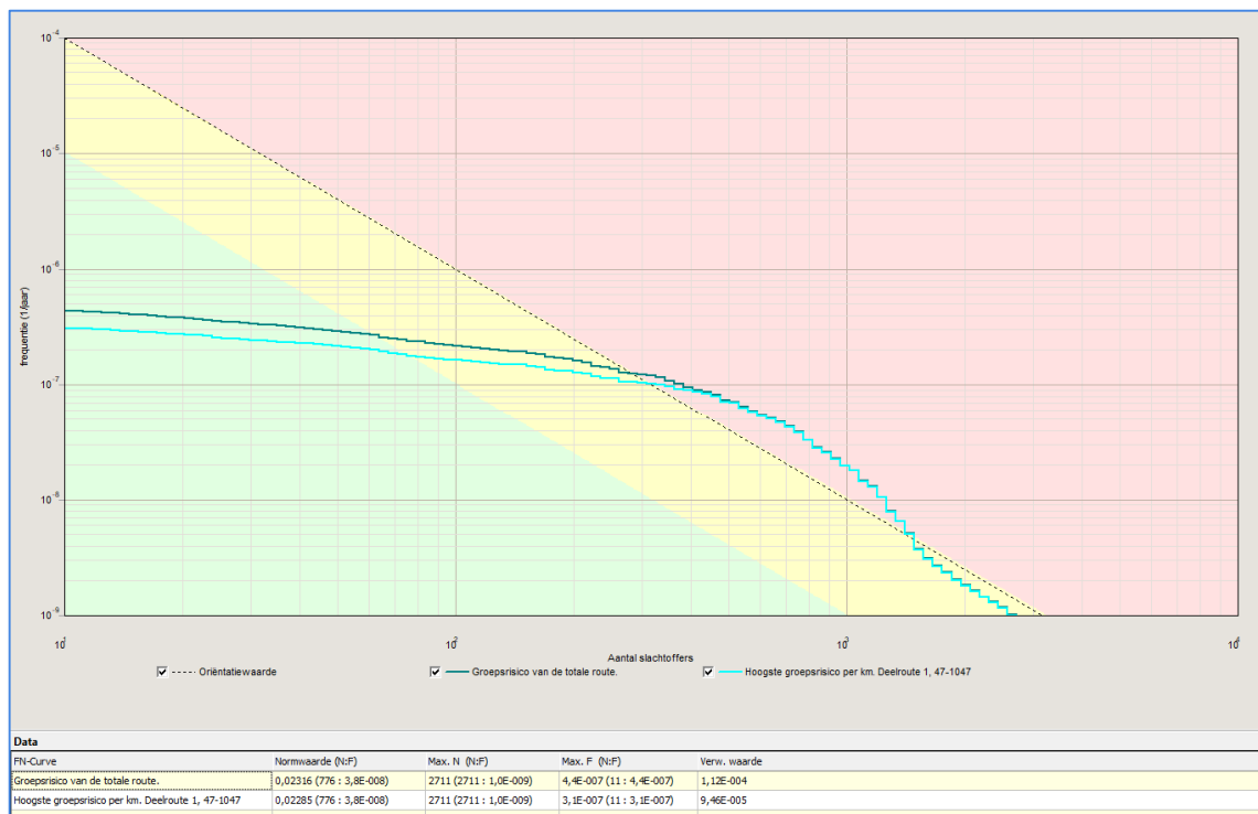
Afbeelding 3 fN-curve berekend groepsrisico, huidige situatie
