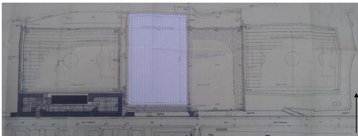
Afbeelding 2.27: Drainage plan van de voetbalvelden met drainagepijpen die om de 3-4 meter zijn aangelegd. Bron: van der Feesten 2012.
