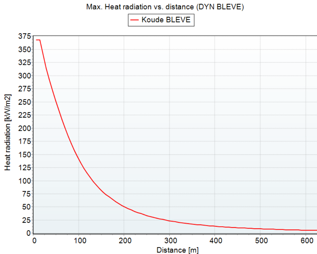
Grafiek hittestraling vs. afstand
