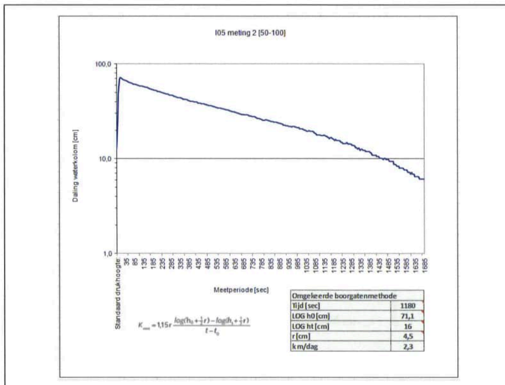
Figuur 14. Infiltratieproef boring B15 (I05), meting 2
