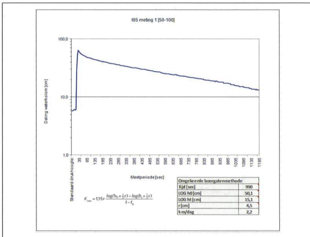
Figuur 13. Infiltratieproef boring B15 (I05), meting 1
