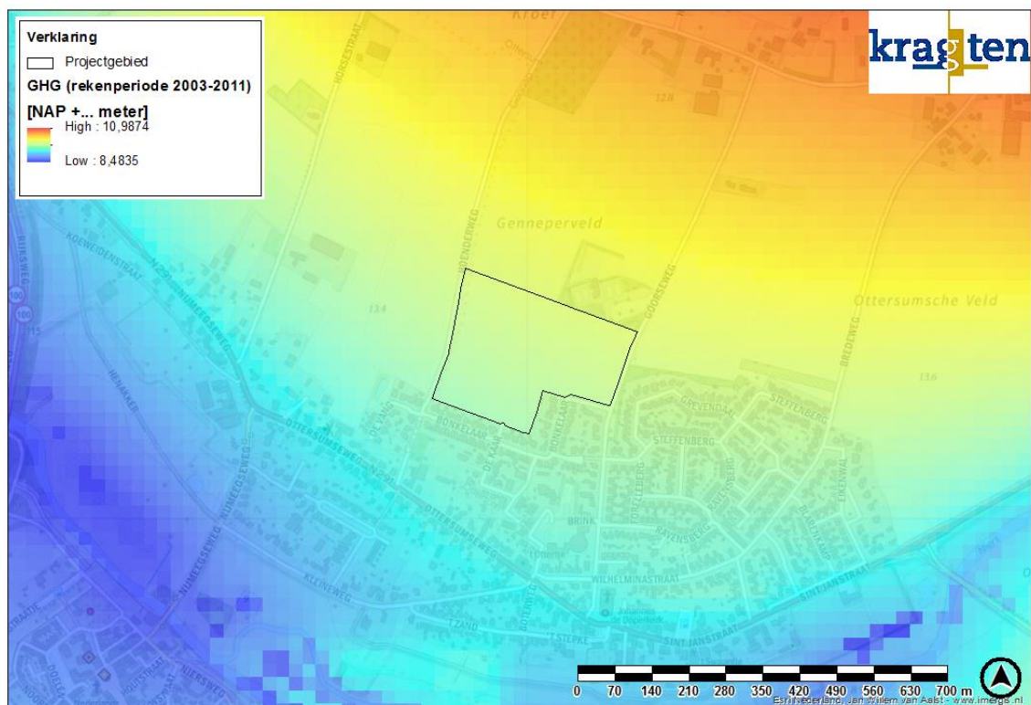
Figuur 8. Grondwaterstanden o.b.v. IBRAHYM resultaten (totale projectgebied fase 1 t/m 5).
