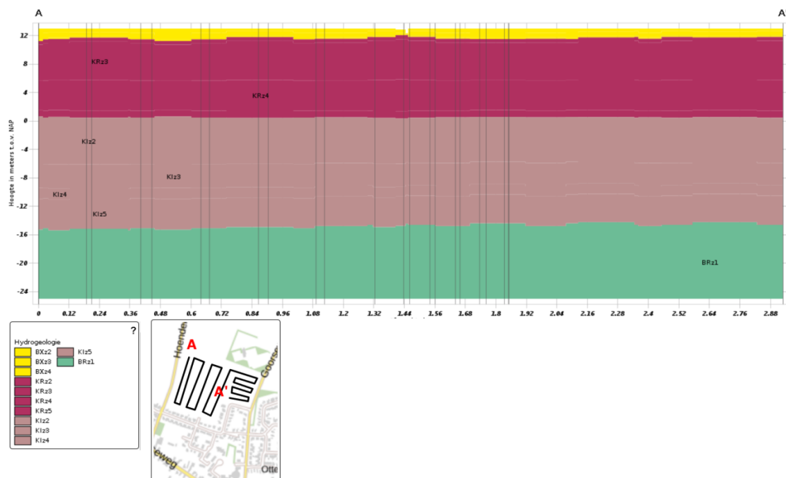
Figuur 6. Geohydrologische doorsnede van de volledige ontwikkeling.
