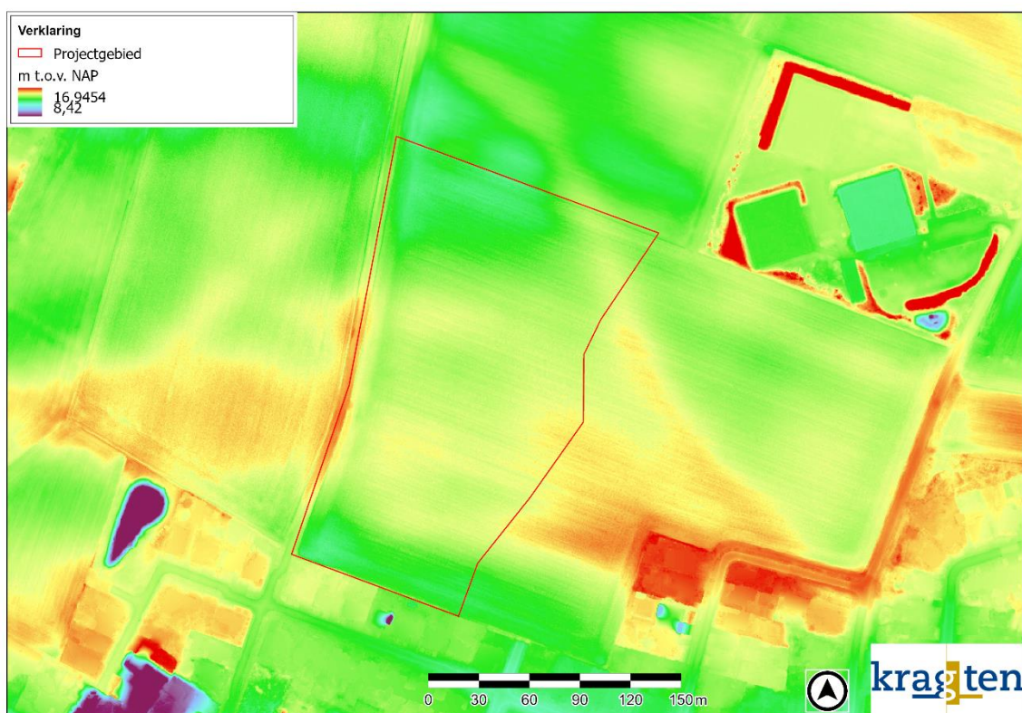
Figuur 5. Maaiveldniveau fase 4 en 5.
