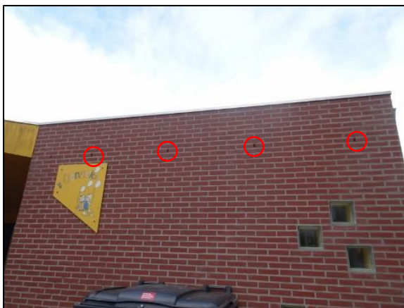
Figuur 11. Open stootvoegen, rood omcirkeld.
