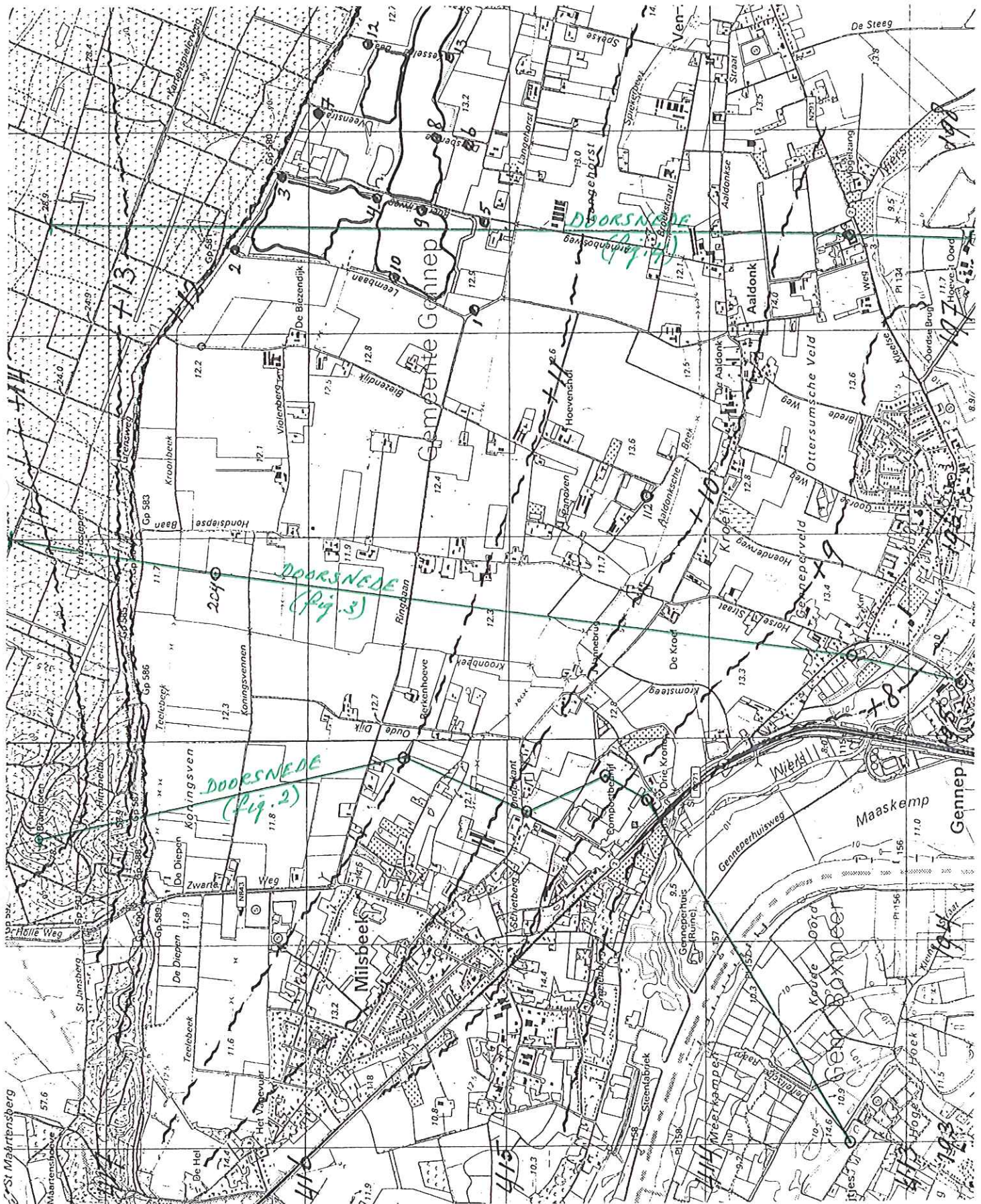
Fig.1; Overzichtskaartje ontgrondingsgebied Koningsven - De Banen met grondwaterishypsen in m. t.o.v. NAP en verloop van de doorsneden; schaal 1:25.000.
