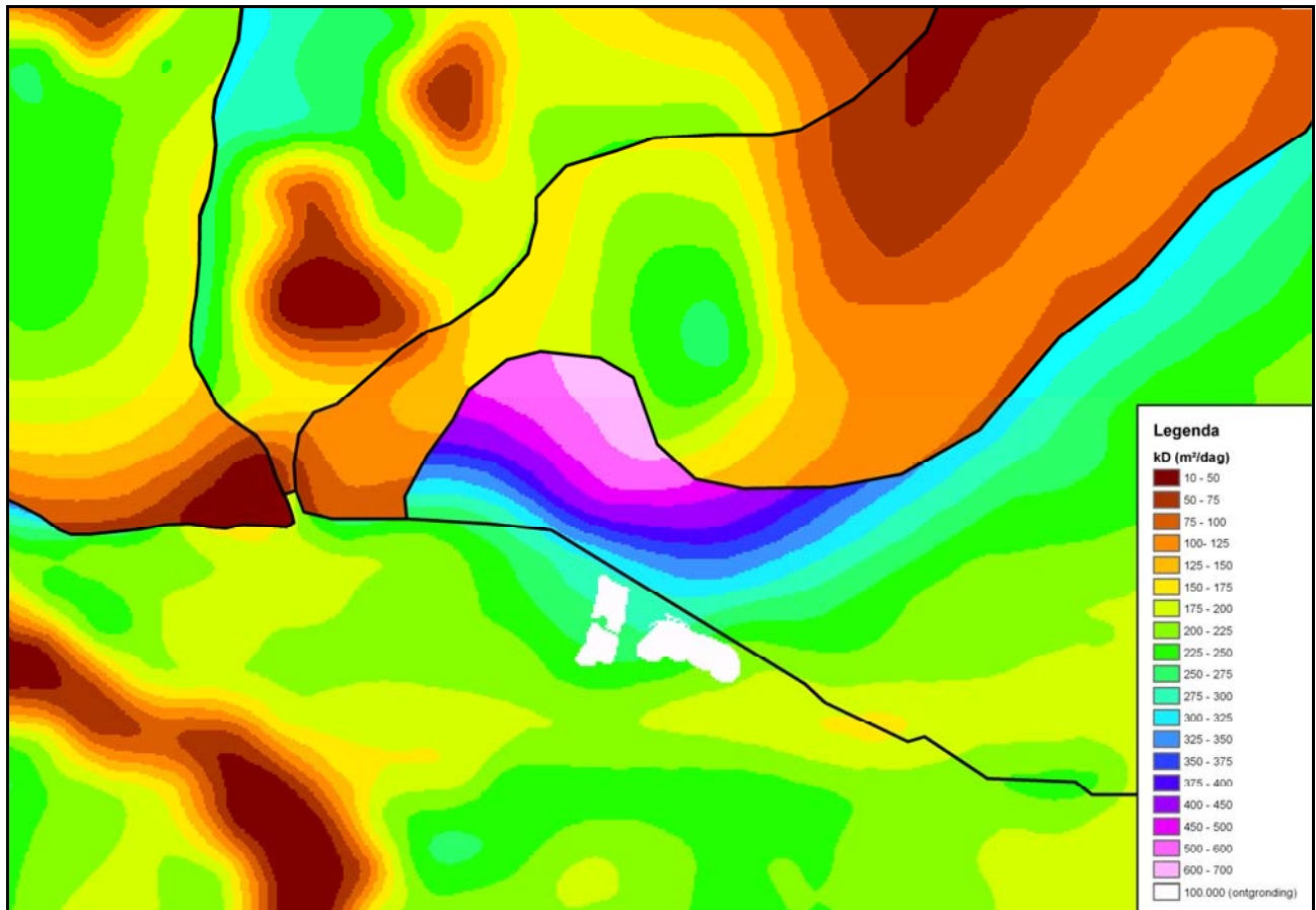
Figuur.1: Doorlaat vermogen (kD) van de bovenste modellaag met de plassen van 'De Banen'.
