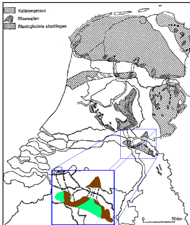
Figuur 2.3: Stuwwallen, keileem en fluvio-glaciale afzettingen (Zonneveld, 1971)
