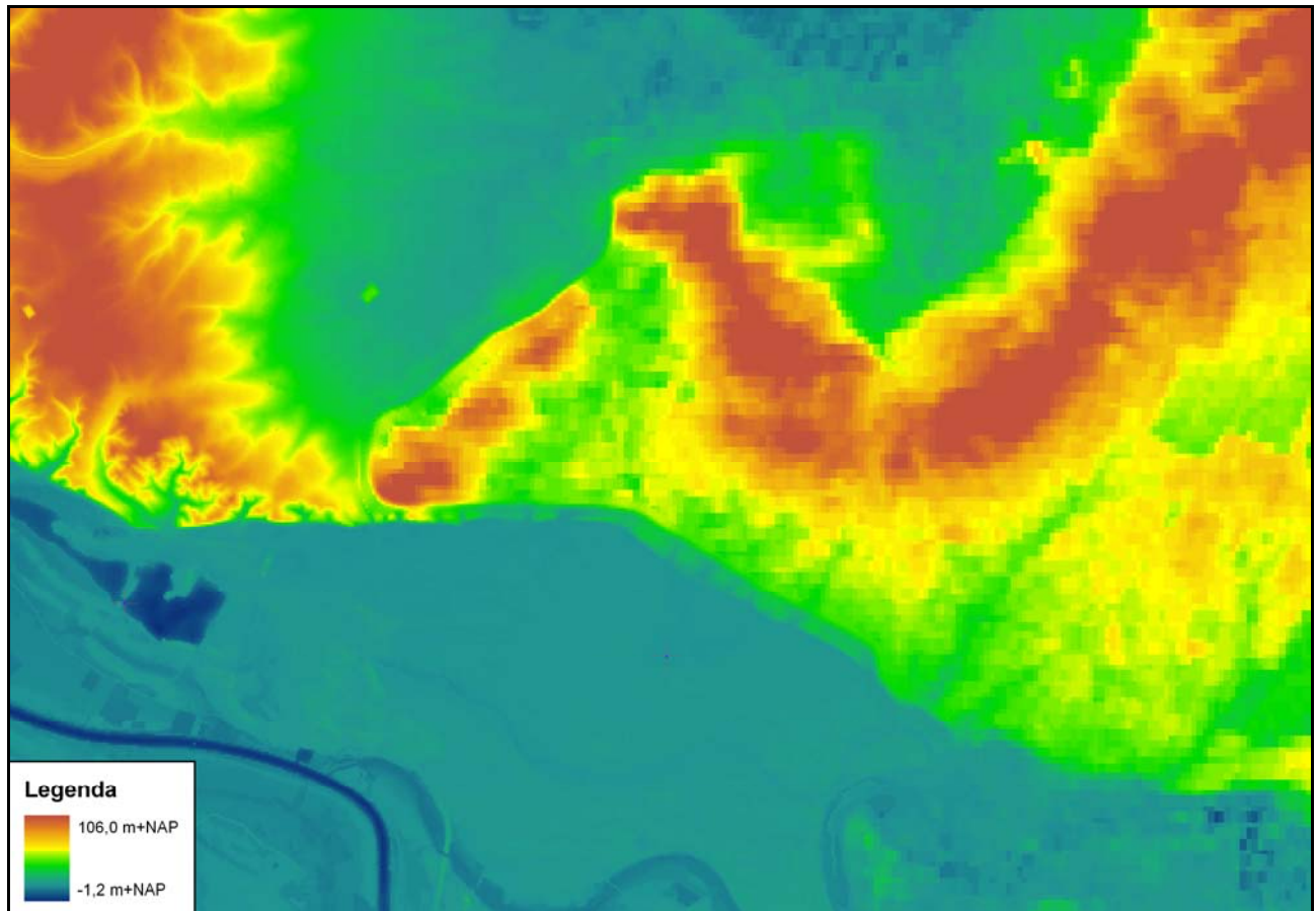
Figuur 2.2: Hoogtekaart van het modelgebied.
