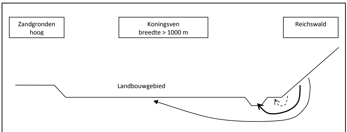
Figuur 2.10: Grondwaterstroom in de actuele situatie (beken dicht bij stuwwal). De gestippelde lijn geeft een korte ondiepe stroombaan en een relatief kleine toevoer van water weer. Naar de Kroonbeek stroomt relatief het meeste water. De stroombaan is gemiddeld langer en weinig dieper. Uit de modelberekeningen voor de referentiesituatie volgt dat weinig water dat onder de beek doorstroomt in het achtergelegen landbouwgebied naar boven komt. De invloed van het neerslagoverschot is hier groter.
