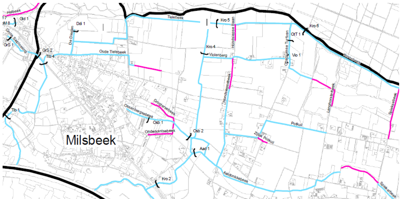
Figuur 2.7: Leggerkaart van de omgeving van het plangebied met in het noordoosten de Kroonbeek, die niet in verbinding staat met de Teelebeek (verticaal streepje). De Kroonbeek voert via stuw Kro 4 af in zuidelijke richting. De Teelebeek voert af in westelijke richting. Blauw zijn de hoofdwatgangen en paars de secundaire watergangen (beide in onderhoud bij het waterschap).
