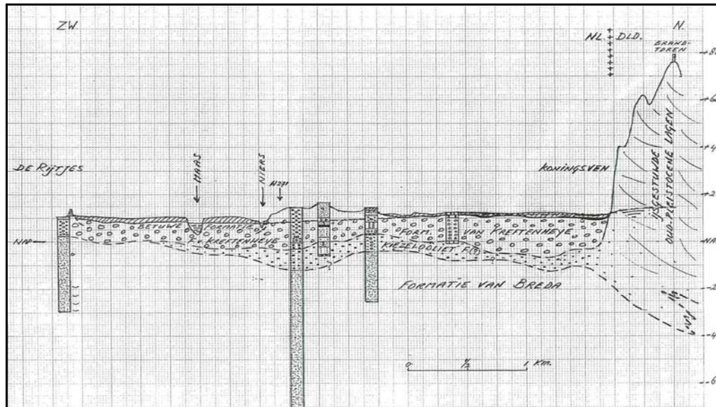
Figuur 2.4: Dwarsdoorsnede geologische opbouw (Van Rooijen 2006, zie bijlage 2)
