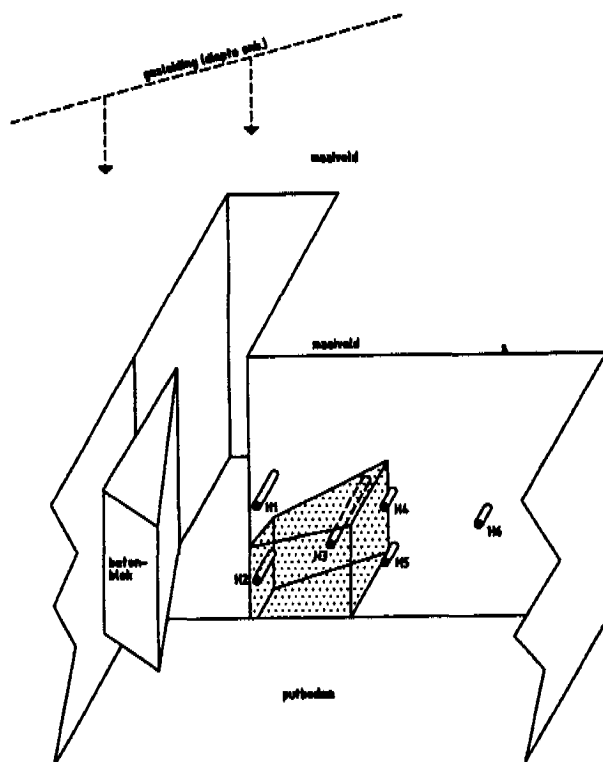
VOORAANZICHT OOSTWAND
