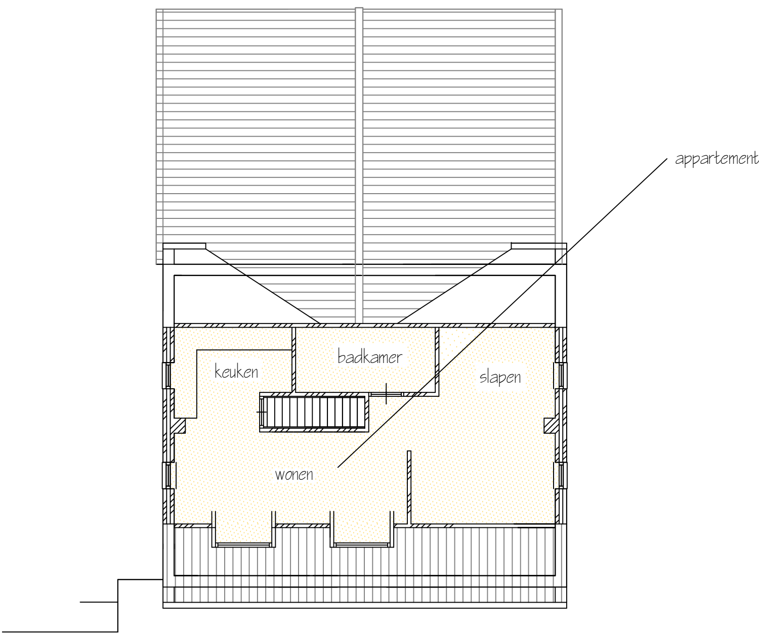
2e verdieping
