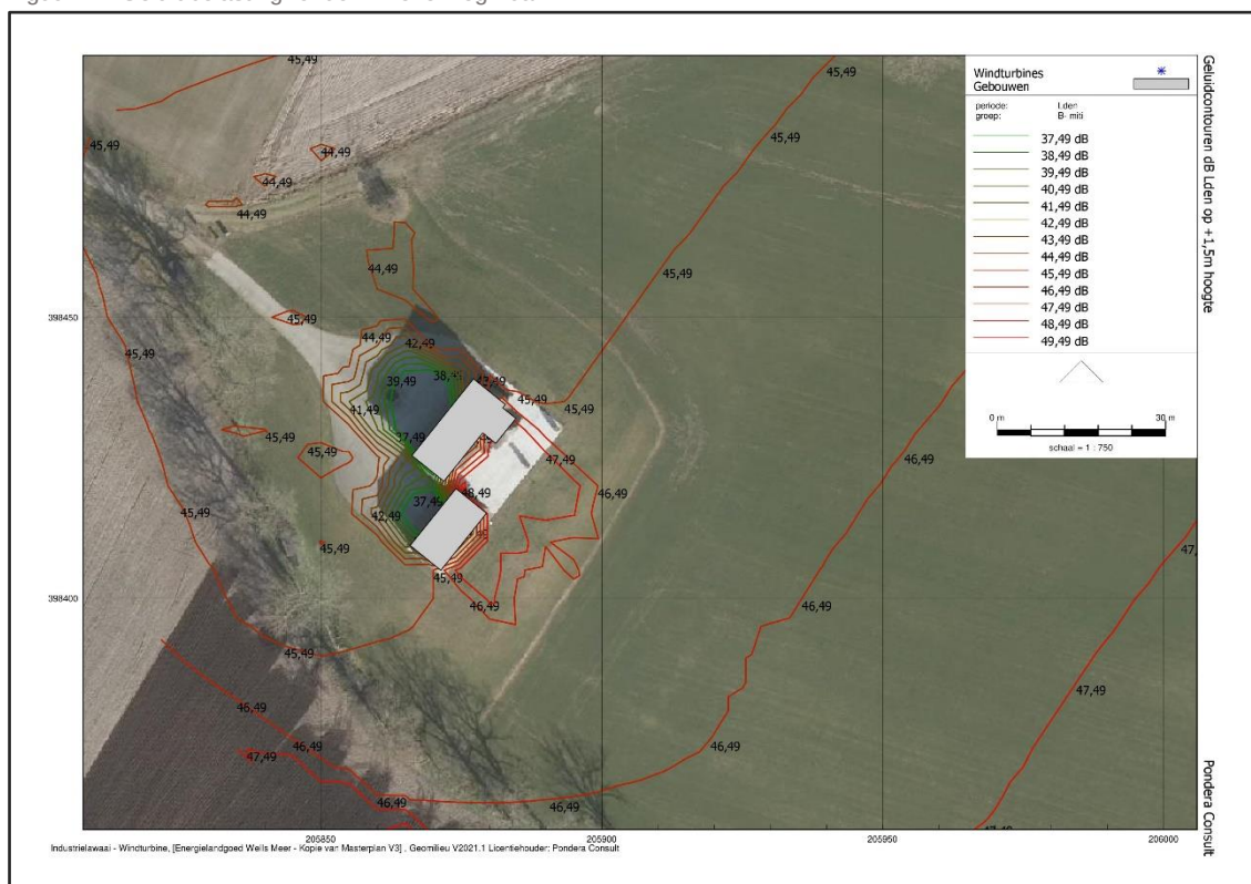
Figuur 1.1 Geluidbelasting rondom Wezerweg 16a
