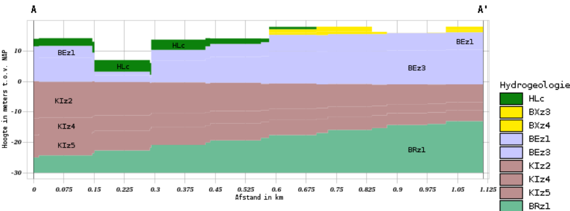
Afbeelding 3: Geohydrologisch model gebaseerd op REGIS II v2.2 (bron 3C)
