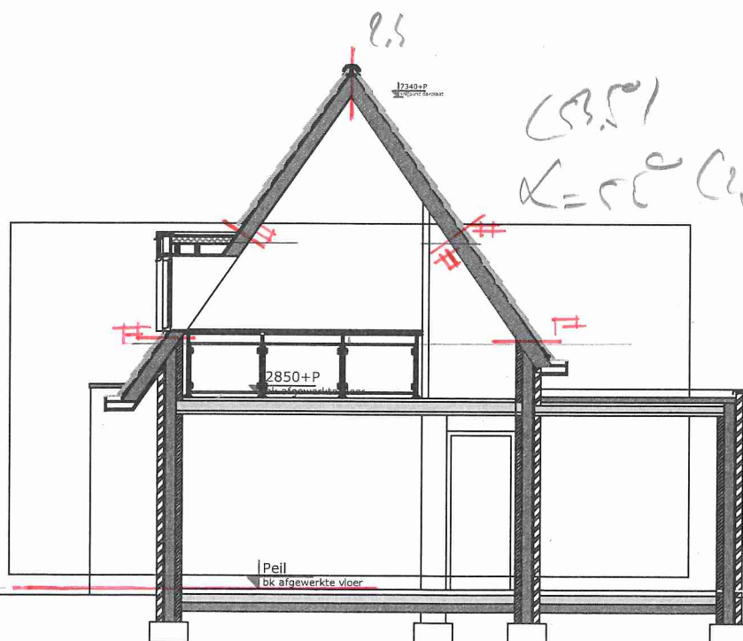
DOORSNEDE A-A
