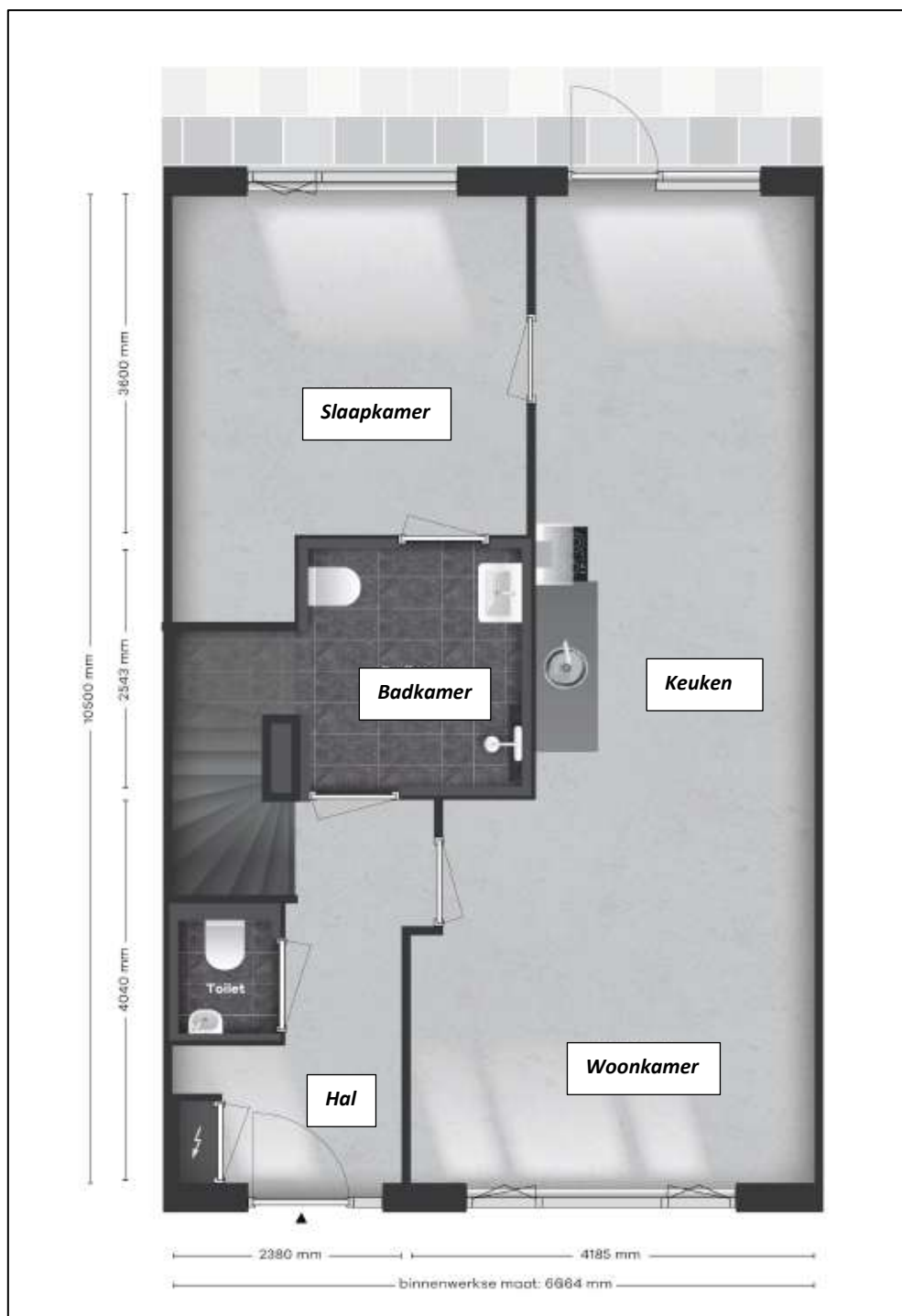
Plattegrond begane grond (bron: MorgenWonen)
