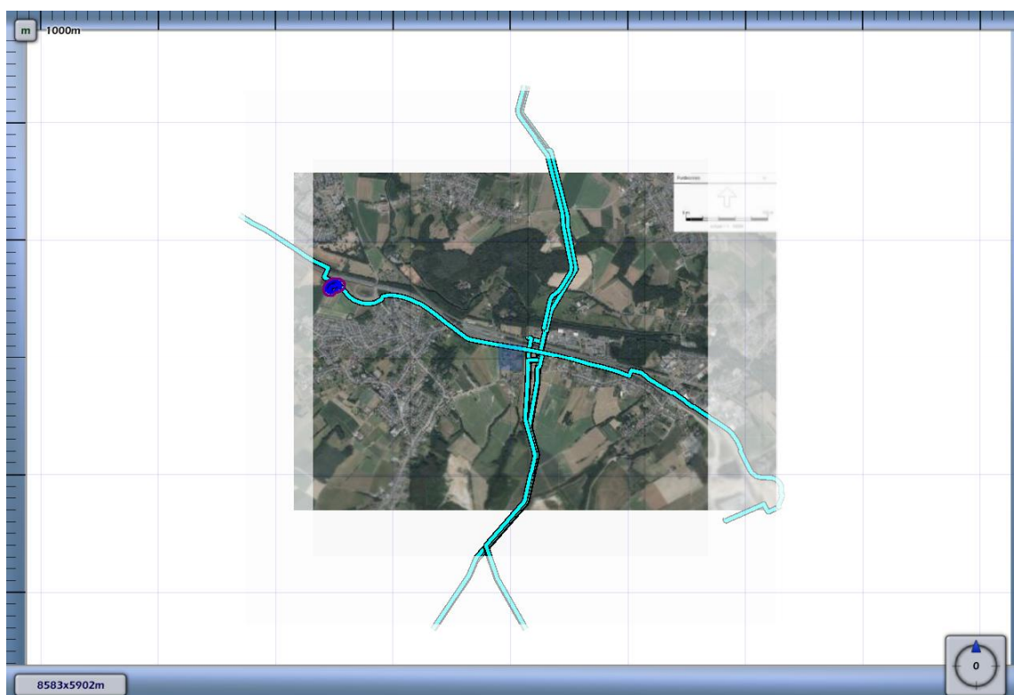
3.11 Figuur 3.11 Plaatsgebonden risico voor 5660_leiding-Z-503-02-deel-1 van N.V. Nederlandse Gasunie
