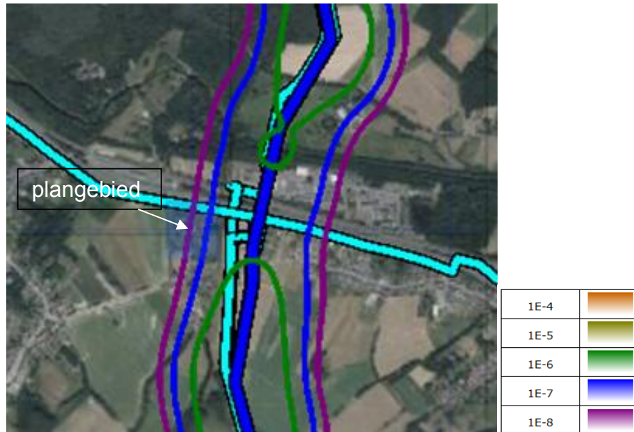
Figuur 2.2: Uitsnede CAROLA plaatsgebonden risico voor leiding A-520-deel-1
