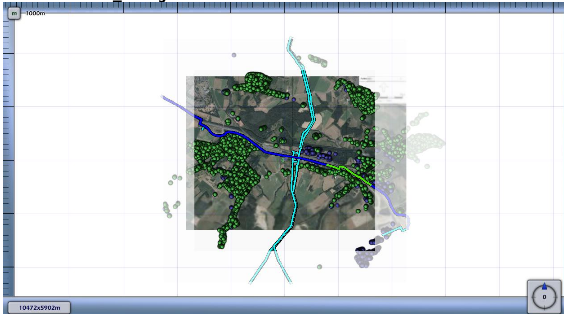
Figuur 4.10 Kilometer leiding behorende bij de maximale overschrijding van de FN-curve voor 5660_leiding-Z-503-01-deel-1 van N.V. Nederlandse Gasunie
