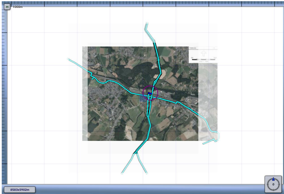
3.5 Figuur 3.5 Plaatsgebonden risico voor 5660_leiding-A-534-deel-1 van N.V. Nederlandse Gasunie
