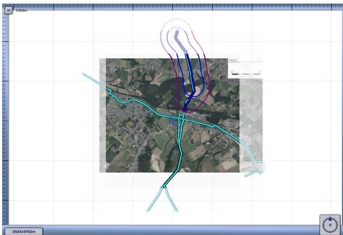
3.7 Figuur 3.7 Plaatsgebonden risico voor 5660_leiding-A-630-deel-1 van N.V. Nederlandse Gasunie
