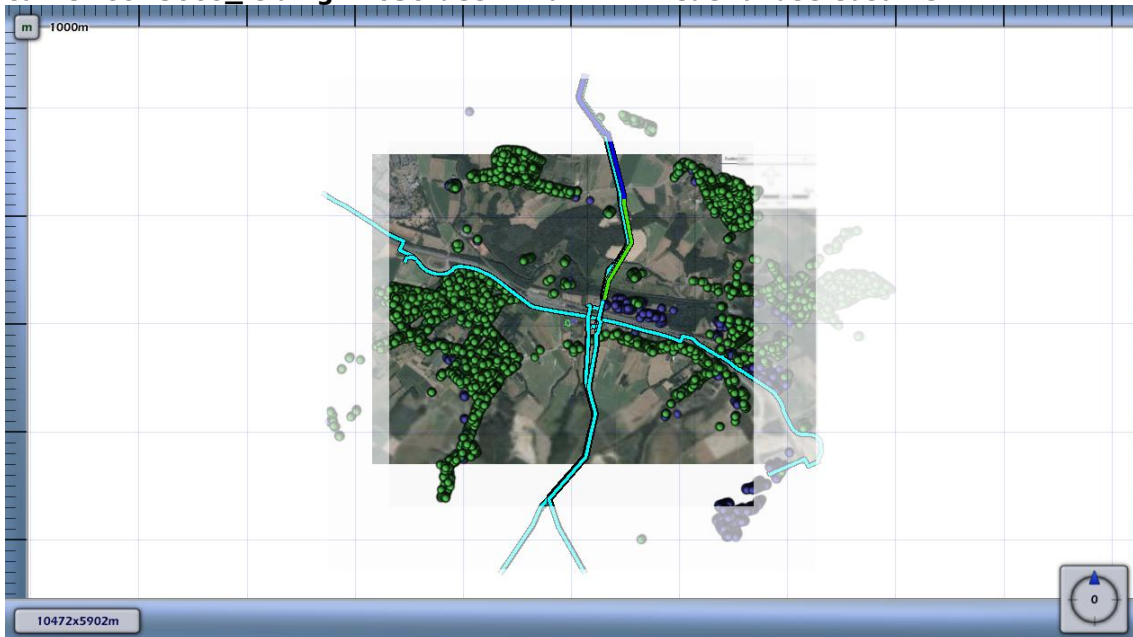
Figuur 4.7 Kilometer leiding behorende bij de maximale overschrijding van de FN-curve voor 5660_leiding-A-630-deel-1 van N.V. Nederlandse Gasunie
