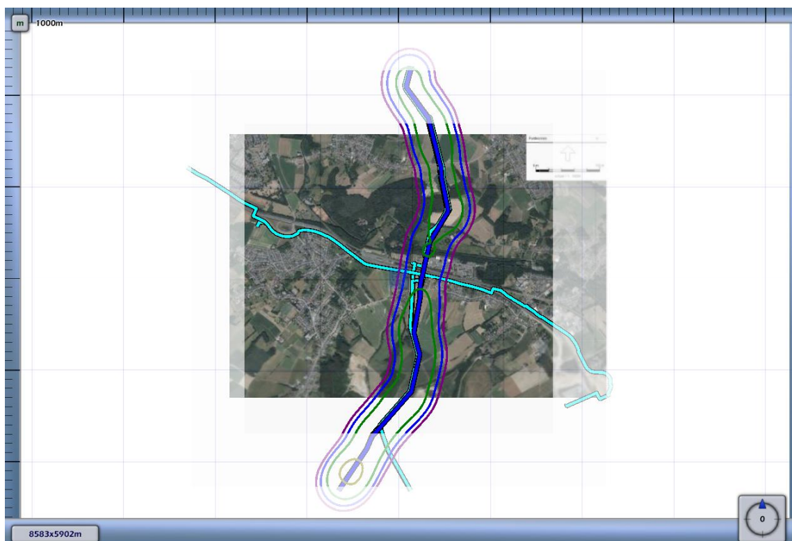
3.1 Figuur 3.1 Plaatsgebonden risico voor 5660_leiding-A-520-deel-1 van N.V. Nederlandse Gasunie
