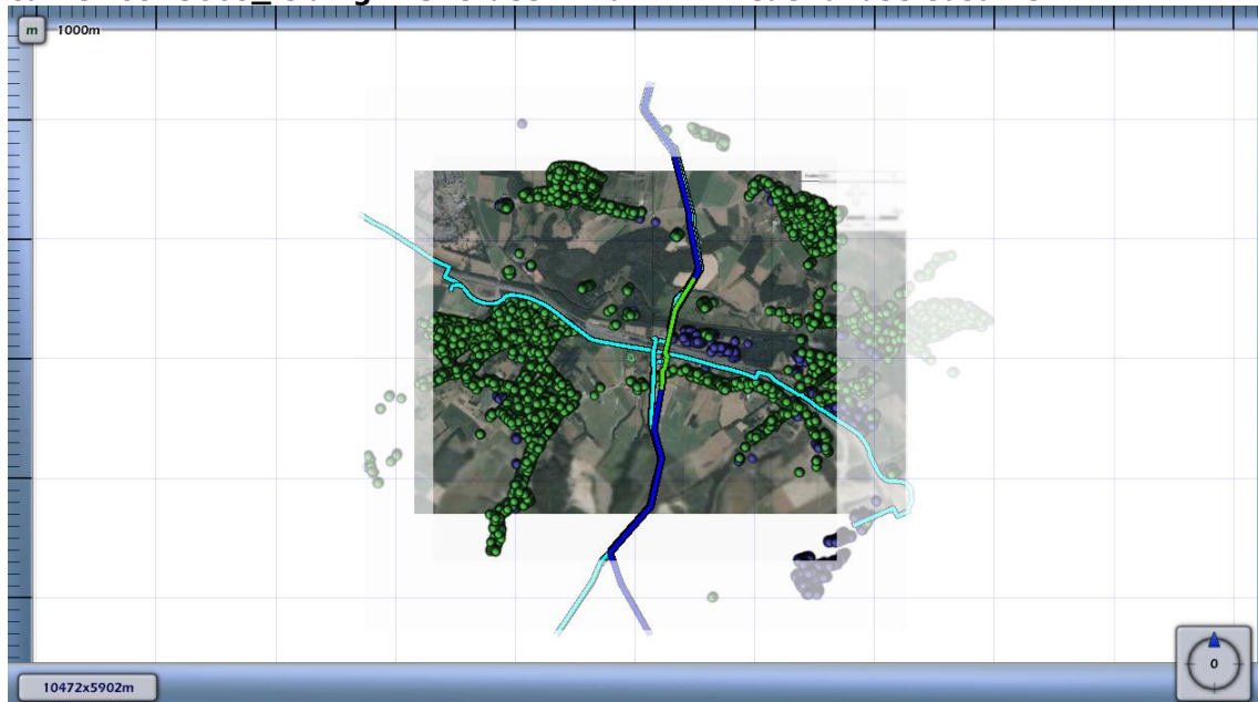
Figuur 4.6 Kilometer leiding behorende bij de maximale overschrijding van de FN-curve voor 5660_leiding-A-578-deel-1 van N.V. Nederlandse Gasunie
