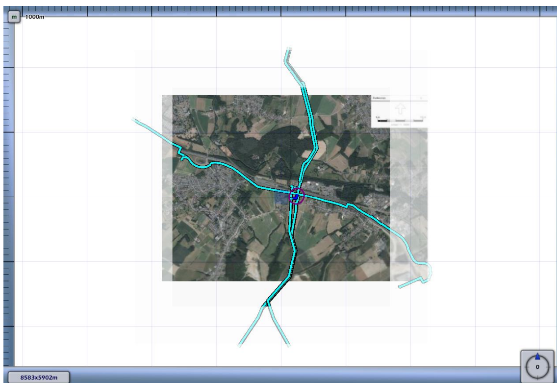
3.13 Figuur 3.13 Plaatsgebonden risico voor 5660_leiding-Z-503-23-deel-1 van N.V. Nederlandse Gasunie
