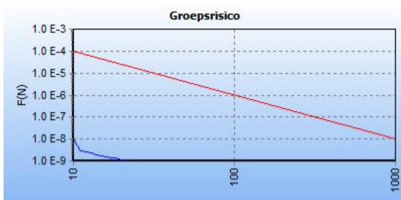
5.10 Figuur 5.10 FN curve voor 5660_leiding-Z-503-01-deel-1 van N.V. Nederlandse Gasunie voor de kilometer tussen stationing 3570.00 en stationing 4570.00
