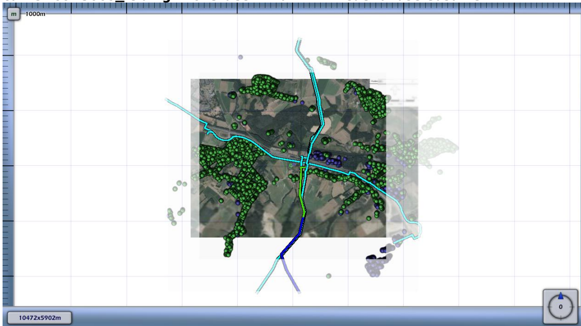
Figuur 4.8 Kilometer leiding behorende bij de maximale overschrijding van de FN-curve voor 5660_leiding-A-645-deel-1 van N.V. Nederlandse Gasunie
