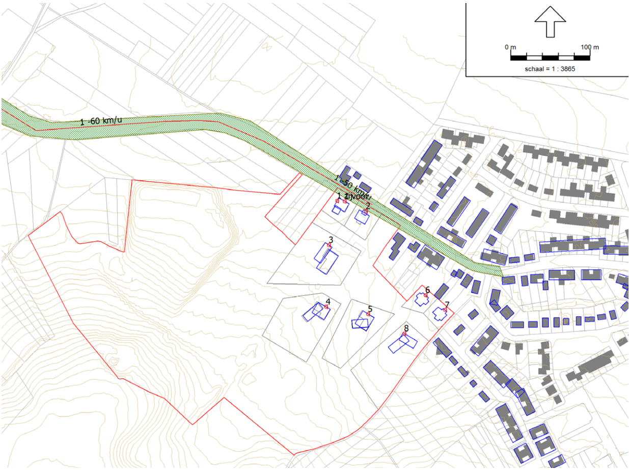
Situatietekening wegverkeerslawaai (Bron: "Akoestisch onderzoek/ Gevelbelasting Loowinkelstraat", Bureau Geluid, 13.06.2013)
