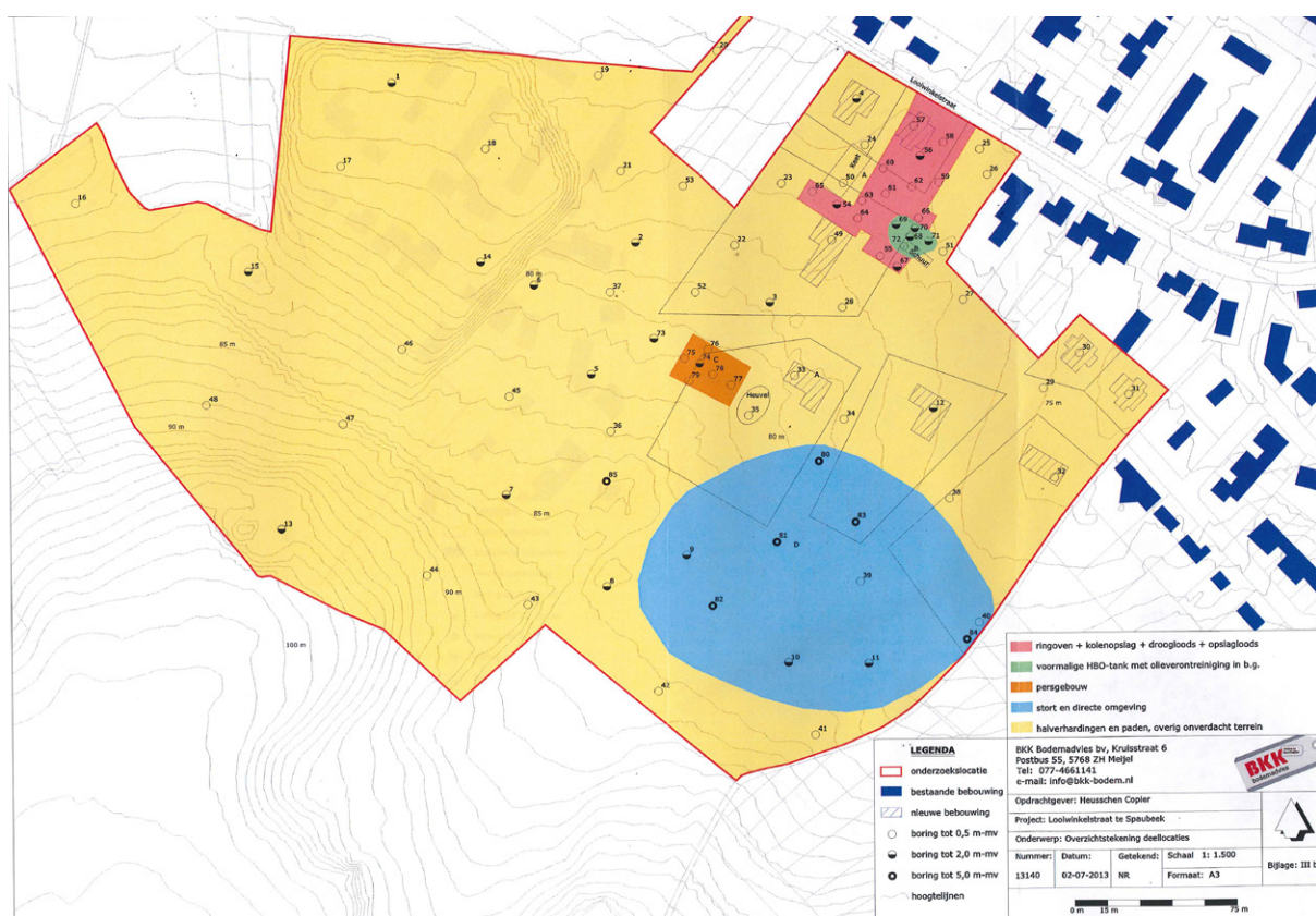
Overzichtstekening bodemonderzoek met boringen
