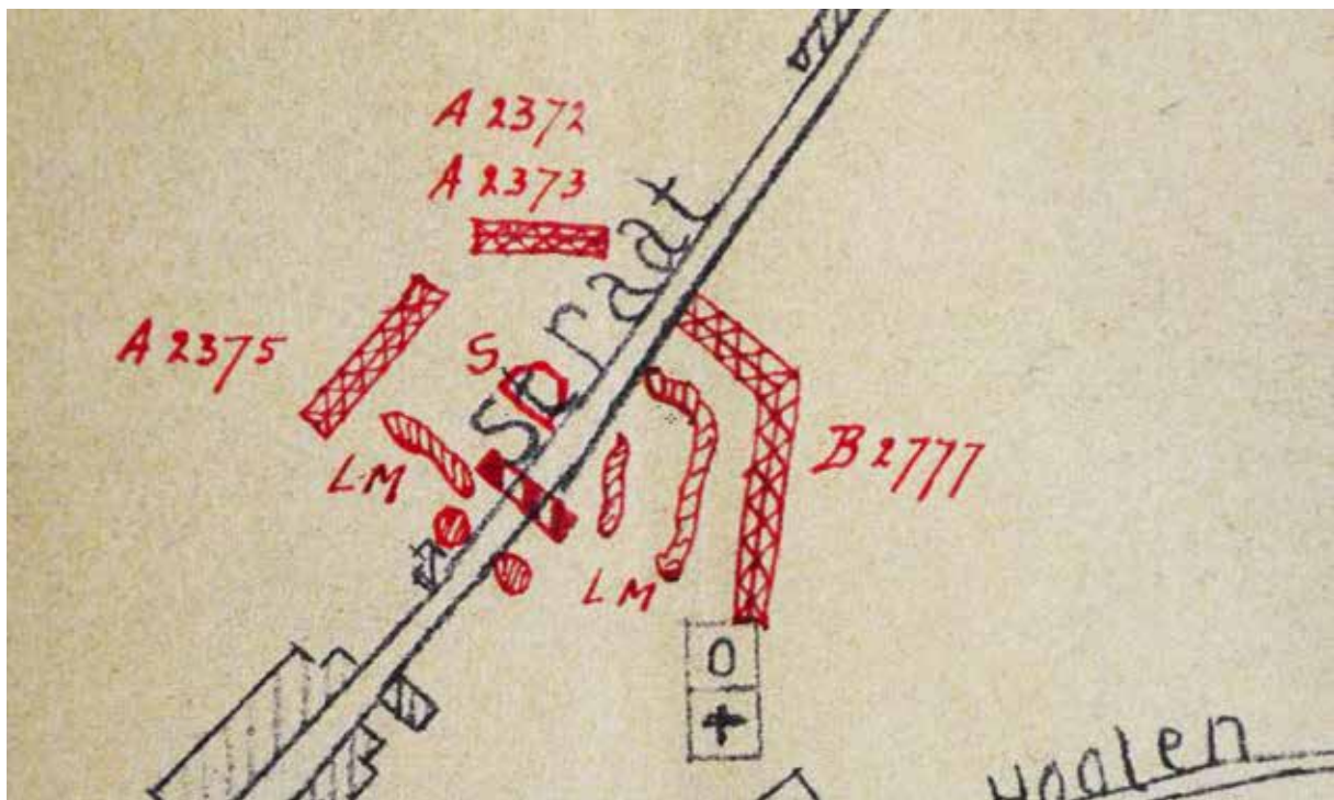
Figuur 4. De verdedigingswerken in de Grensstraat, een van de drie onderdelen van Object Waubach. Bron: NIMH, toeg. nr. 405, inv. nr. 24 II-10.
