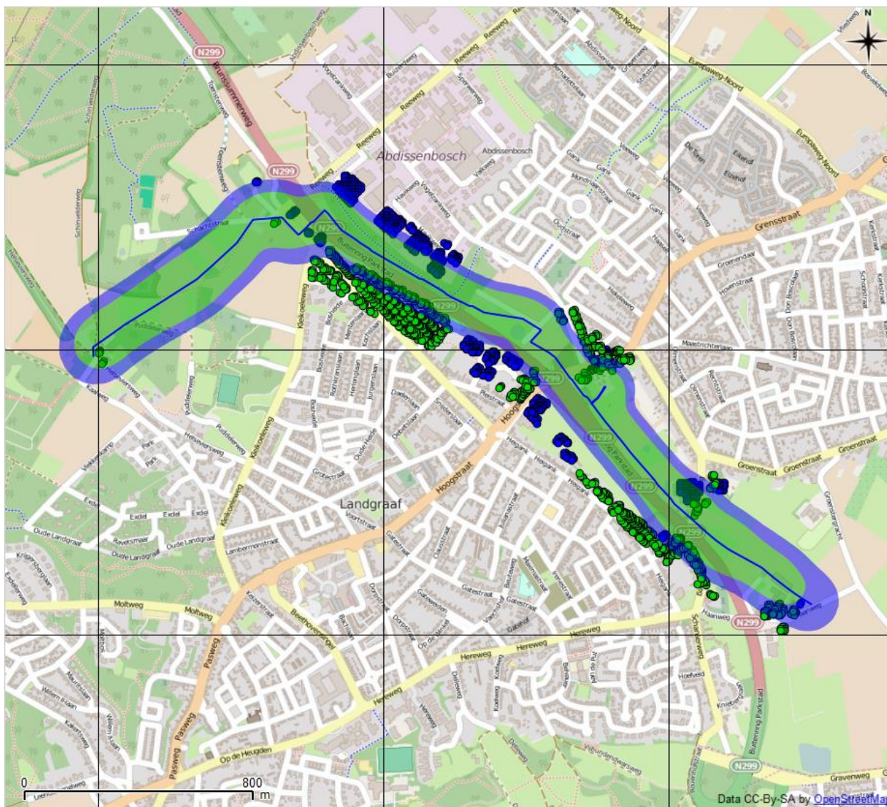
Figuur 4 Ligging van gastransportleiding Z-503-01 (donkerblauw) in de toekomstige situatie. De plaatsgebonden risicocontouren rondom de leiding zijn, wanneer aanwezig, weergegeven met de volgende kleuren:
