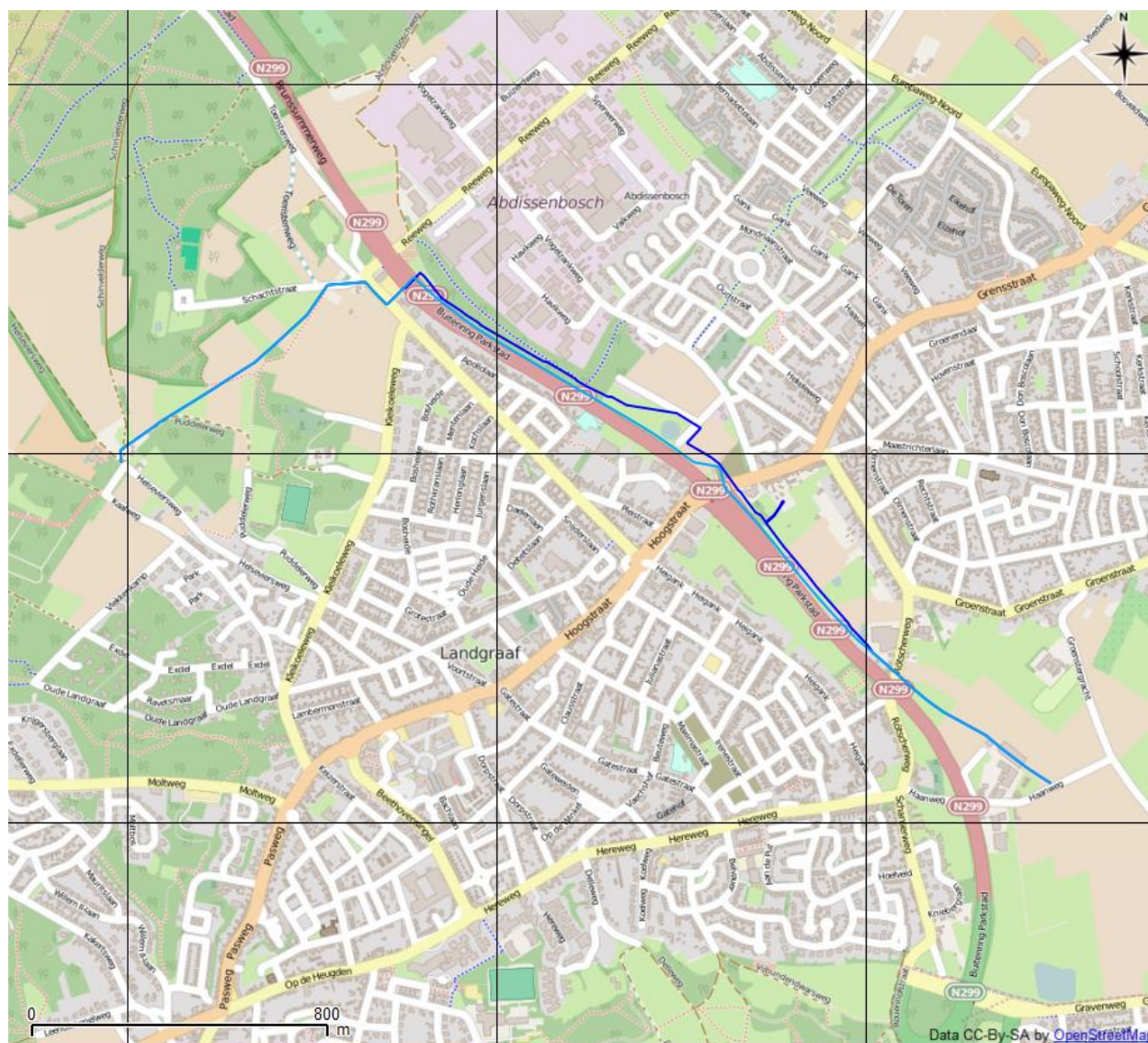
Figuur 1 Ligging van gastransportleiding Z-503-01. De ligging van de leiding in de huidige situatie is weergegeven in het lichtblauw en de verlegging in het donkerblauw.
