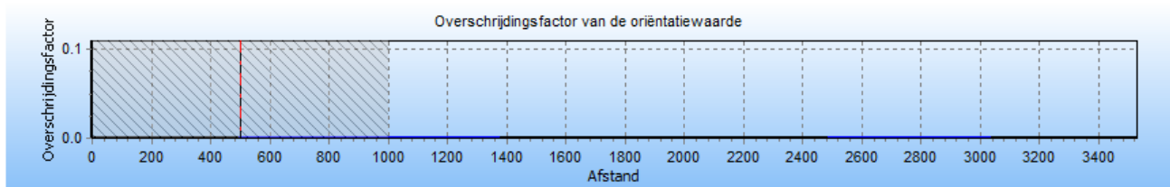
Figuur 7 Overschrijding van het groepsrisico als functie van de stationing van de Z-503-01.
