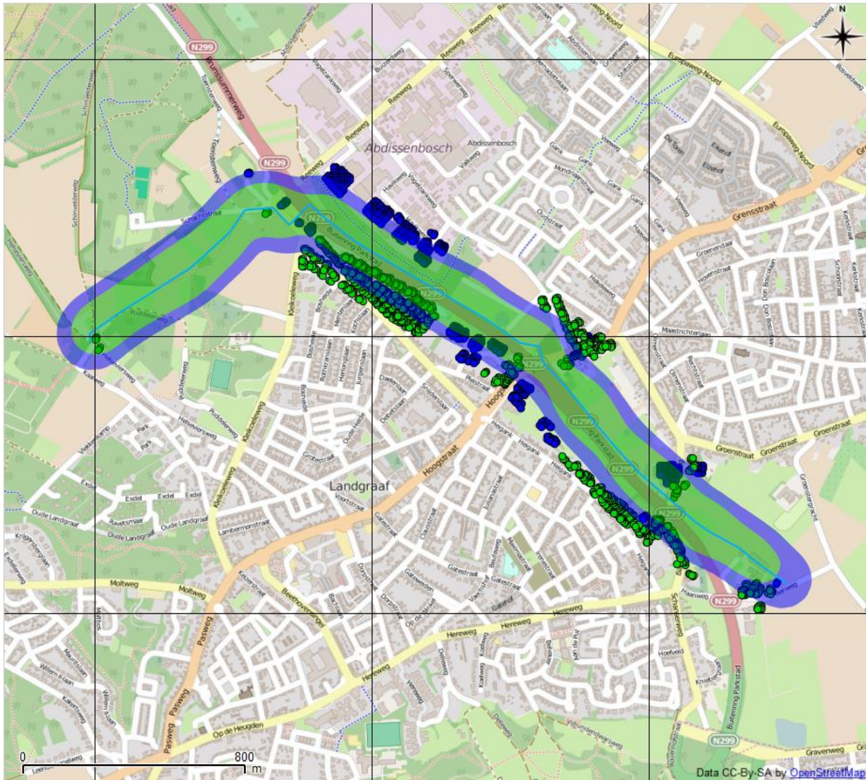
Figuur 3 Ligging van gastransportleiding Z-503-01 (lichtblauw) in de huidige situatie. De plaatsgebonden risicocontouren rondom de leiding zijn, wanneer aanwezig, weergegeven met de volgende kleuren:
