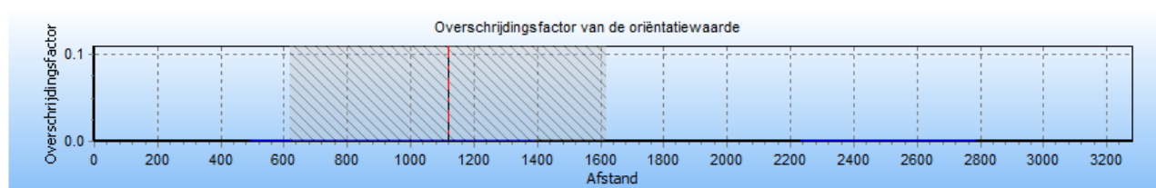
Figuur 5 Overschrijding van het groepsrisico als functie van de stationing van de Z-503-01.
