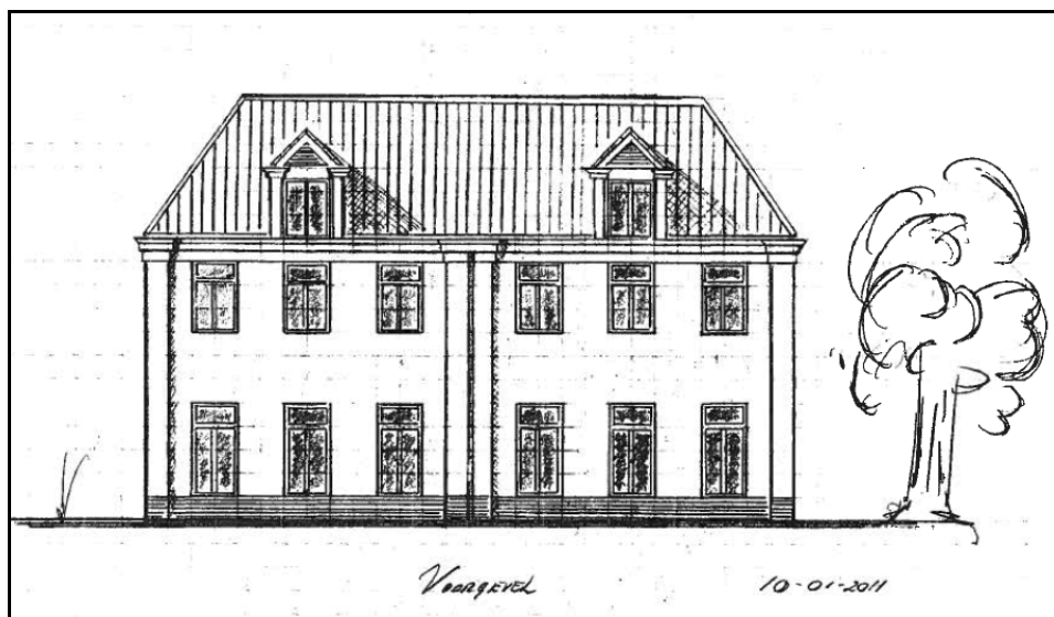
Schets voorgevel
