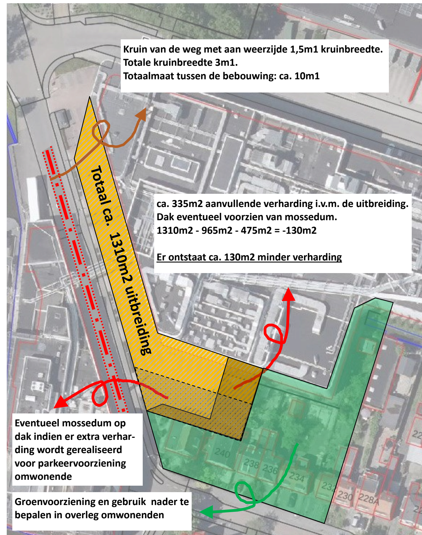
SITUATIE NA UITBREIDING
