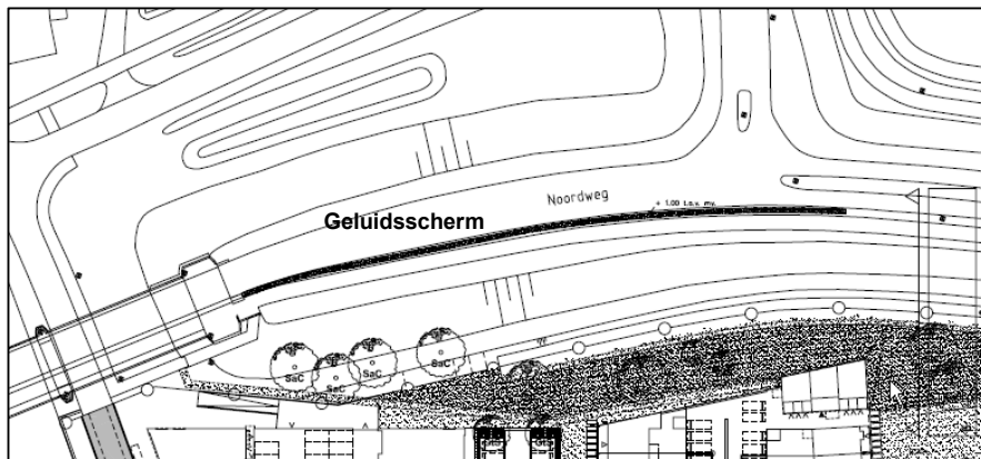
Figuur 5.5: Bovenaanzicht te plaatsen geluidsscherm (bron: Parteon)
