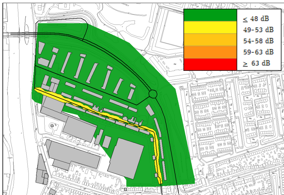
Figuur 5.3: Geluidscontouren Knollendammerstraat (inclusief correctiefactor) bij toepassing asfalt
