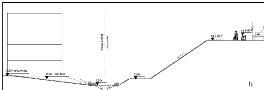
Figuur 5.6: Dwarsdoorsnede van geluidsscherm (bron: Parteon)
