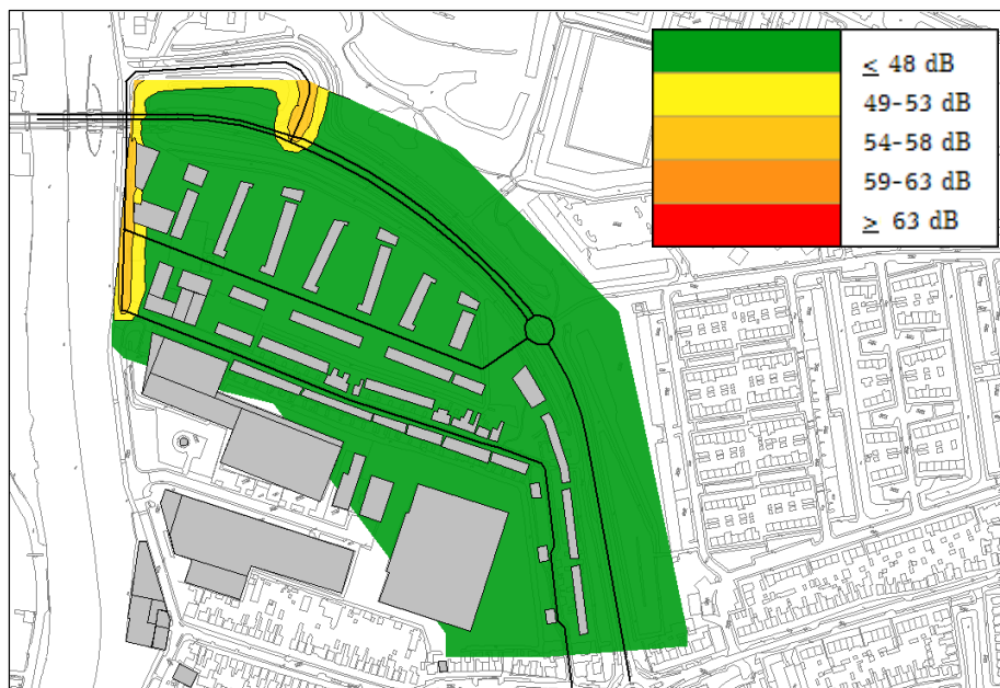
Figuur 5.2: Geluidscontouren Veerdijk (inclusief correctiefactor) bij toepassing geluidreducerend asfalt
