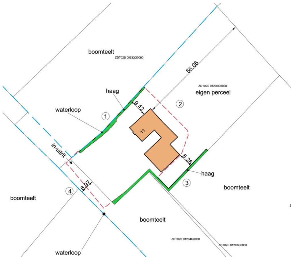
Figuur 14: overzichtstekening
