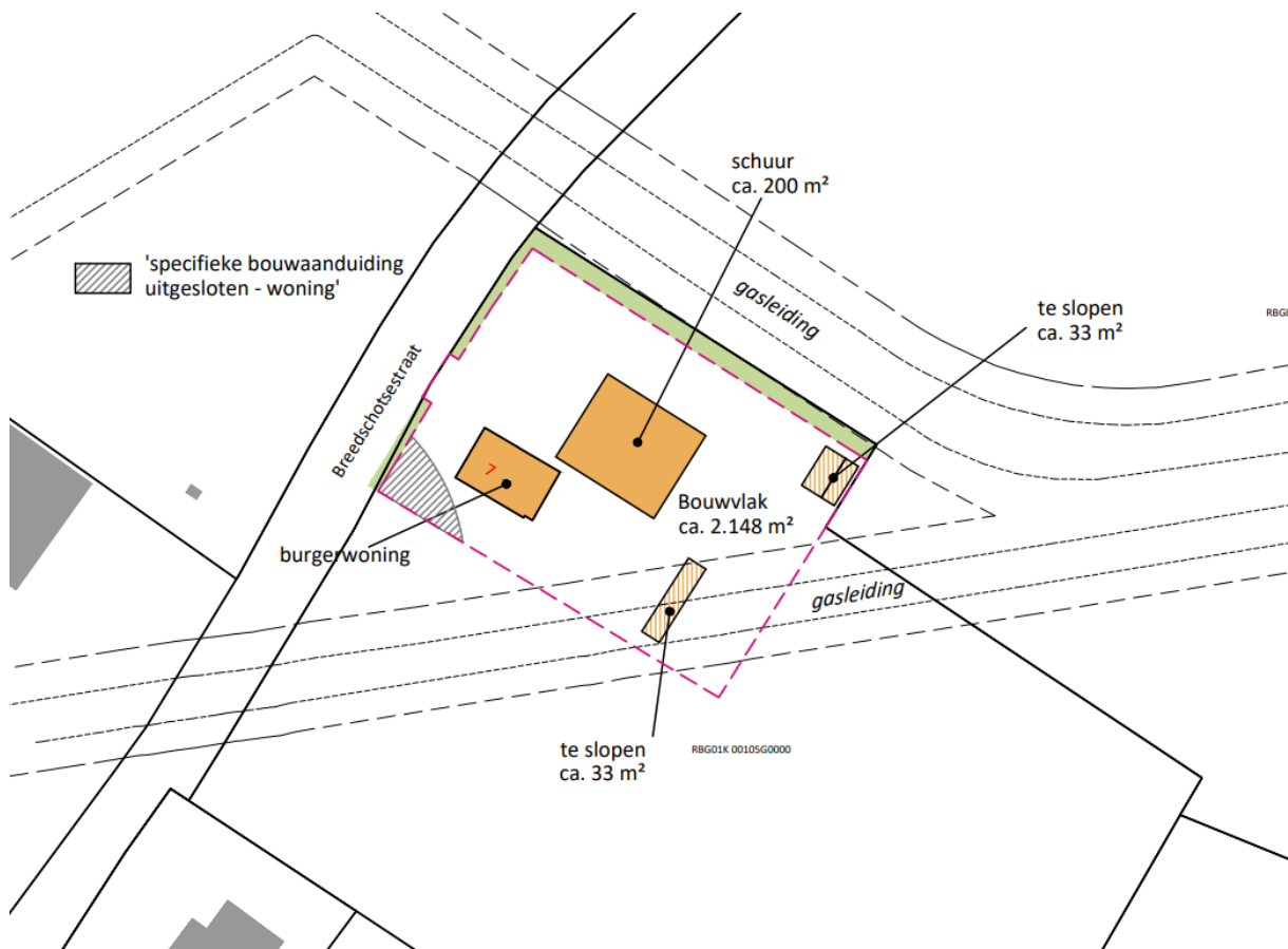
Figuur 6: Nieuwe situatie Breedschotsestraat 7
