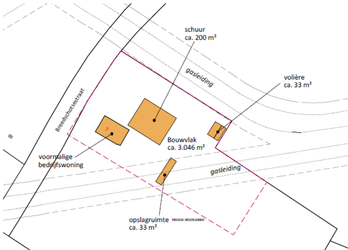
Figuur 5: Overzicht bestaande situatie Breedschotsestraat 7
