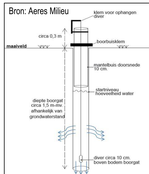
Afbeelding 6: Principetekening meetproef
