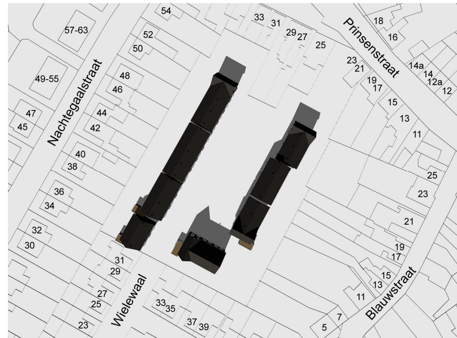
boven : bezonningsdiagram, nieuwe situatie op 21 maart 14.00 uur
