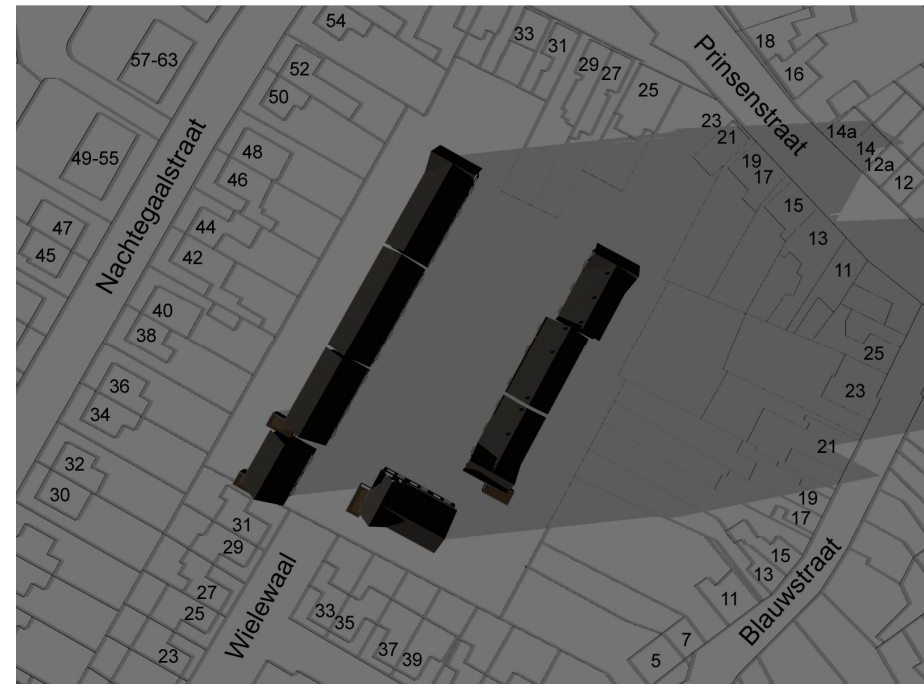
boven : bezonningsdiagram, nieuwe situatie op 21 september 18.00 uur
