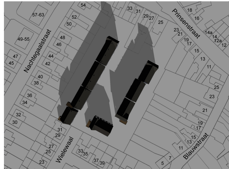
boven : bezonningsdiagram, nieuwe situatie op 21 december 12.00 uur
