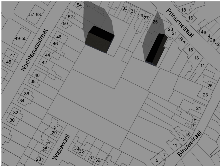
boven : bezonningsdiagram, bestaande situatie op 21 december 12.00 uur
