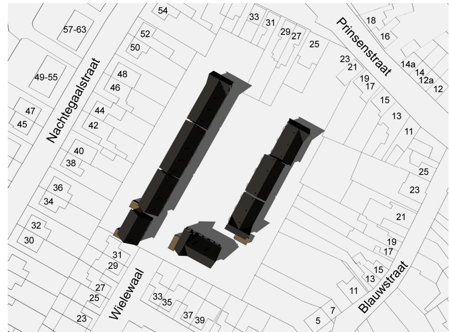
boven : bezonningsdiagram, nieuwe situatie op 21 juni 16.00 uur
