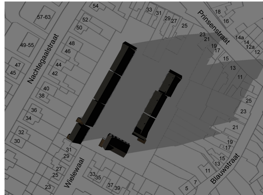
boven : bezonningsdiagram, nieuwe situatie op 21 maart 18.00 uur
