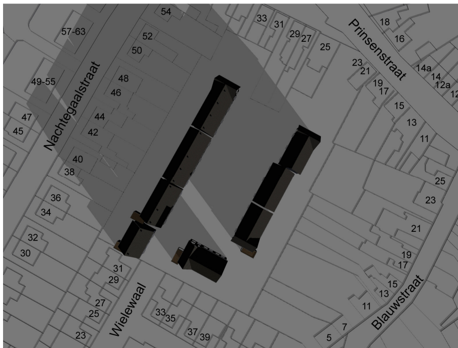
boven : bezonningsdiagram, nieuwe situatie op 21 december 10.00 uur
