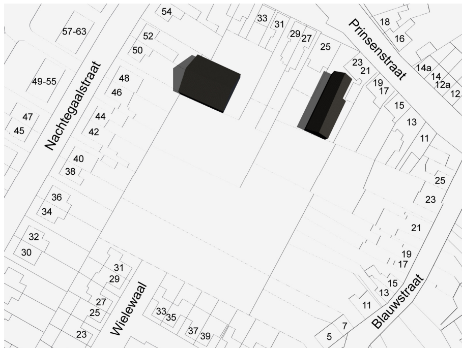
boven : bezonningsdiagram, bestaande situatie op 21 juni 10.00 uur
