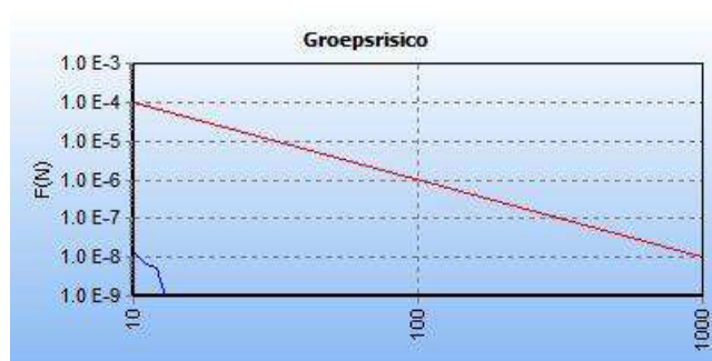
Figuur 3. Groepsrisico A-530 (zowel huidig als toekomstig)
