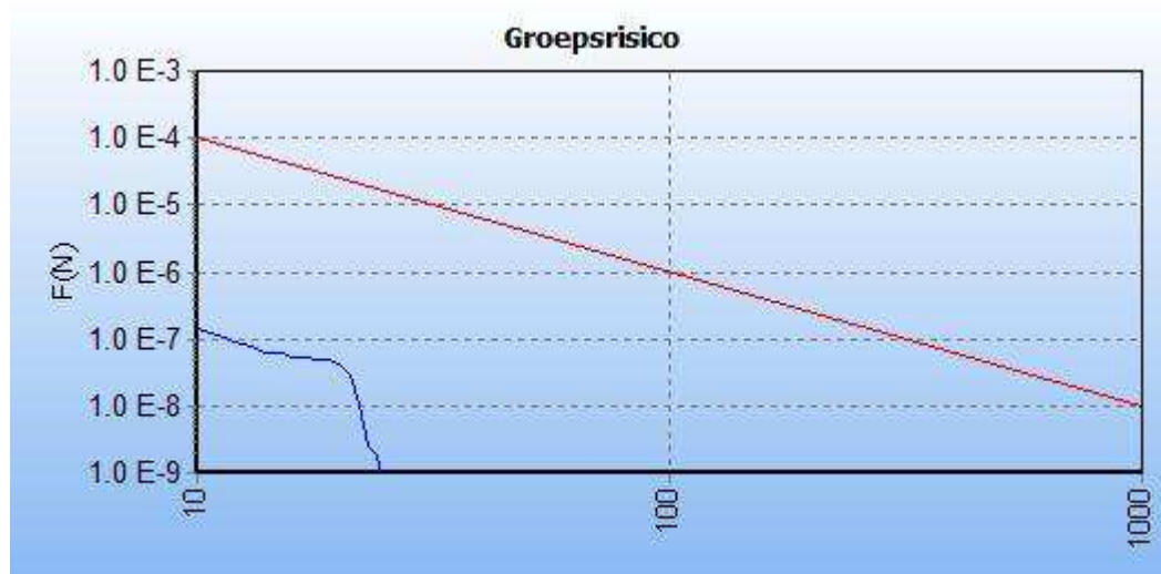
Figuur 5.2 FN curve voor 2901_leiding-A-614-deel-1 van N.V. Nederlandse Gasunie voor de kilometer tussen stationing 1660.00 en stationing 2660.00
