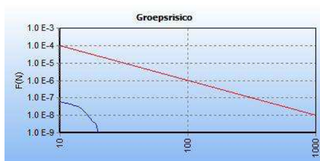
Figuur 4. Groepsrisico A-614 (zowel huidig als toekomstig)
