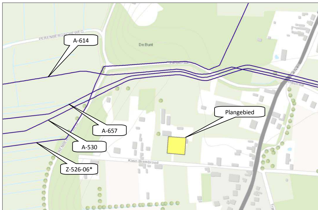
Figuur 1. Plangebied/bouwvlak woning Klein Brembrood Calfven en hogedruk aardgasleidingen
