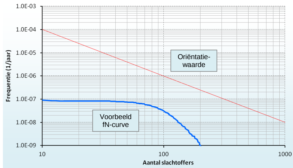
Figuur 8. Voorbeeld groepsrisico aardgasleiding
