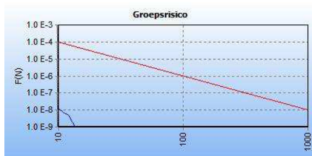
Figuur 5. Groepsrisico A-657 (zowel huidig als toekomstig)
