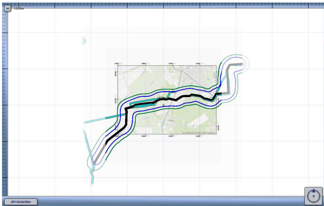
Figuur 3.3 Plaatsgebonden risico voor 2901_leiding-A-657-deel-1 van N.V. Nederlandse Gasunie
