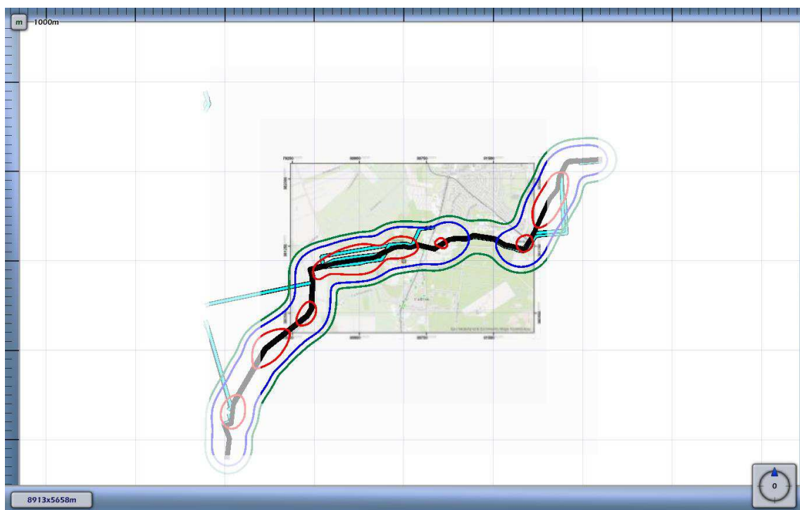
Figuur 3.1 Plaatsgebonden risico voor 2901_leiding-A-530-deel-1 van N.V. Nederlandse Gasunie
