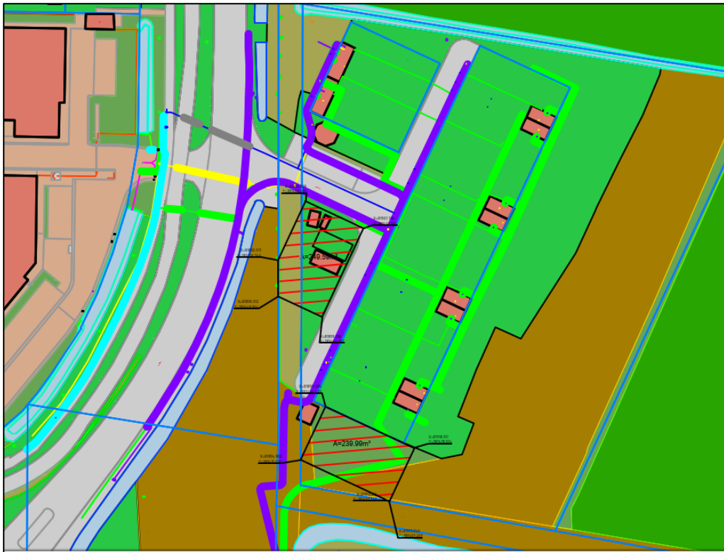
Situatietekening inclusief uitbreidingen aan west- en zuidzijde van het bestaande woonwagencentrum.
