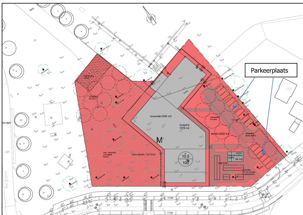
Figuur 2.2: Bouwplan IKC te Woensdrecht.
