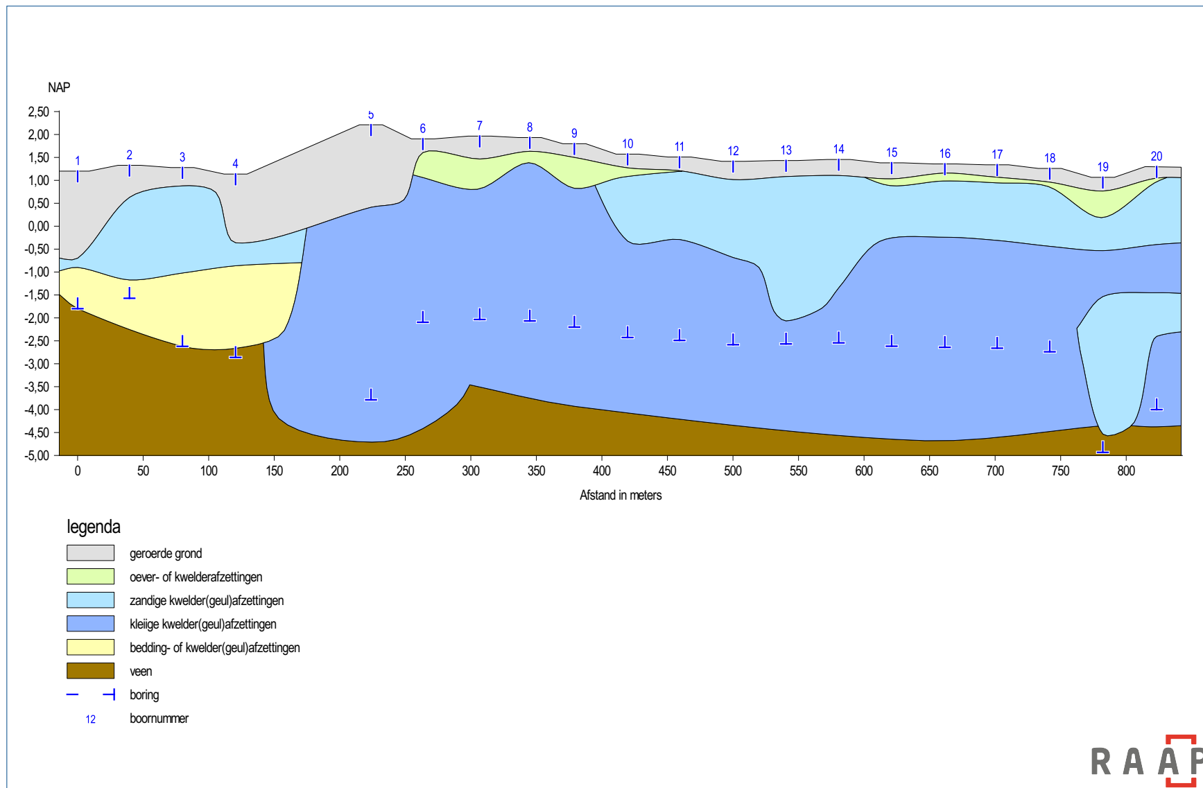
Figuur 3. Dwarsprofiel.
