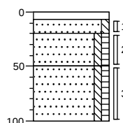
Boring: C06
