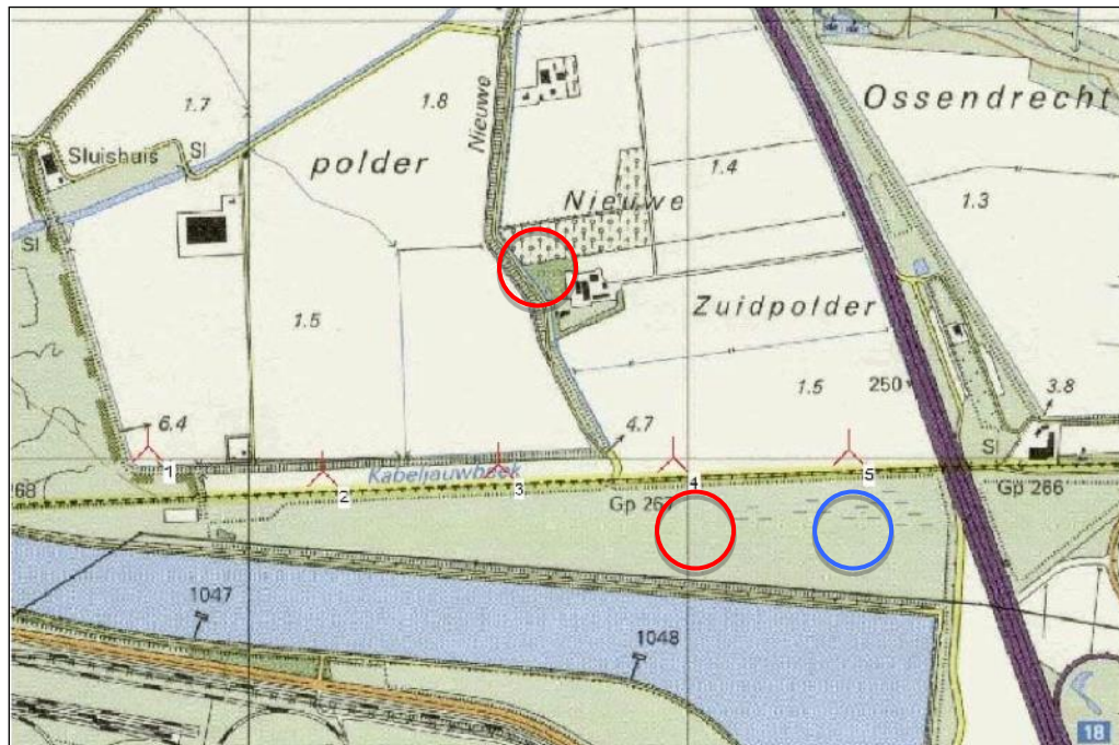
Figuur 3.1 Nestplaatsen buizerd (rode cirkels) en locatie van baltsend paartje bruine kiekendief (blauwe cirkel) in de omgeving van het plangebied Windpark Kabeljauwbeek (op basis van waarnemingen 7 april 2014).
