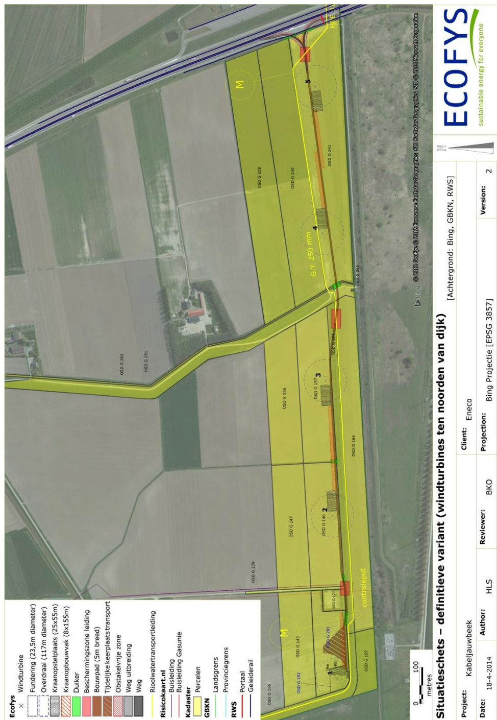
Figuur 2.1 Locaties van de vijf geplande windturbines langs de Kabeljauwbeek ten westen van de A4 in de gemeente Woensdrecht.
