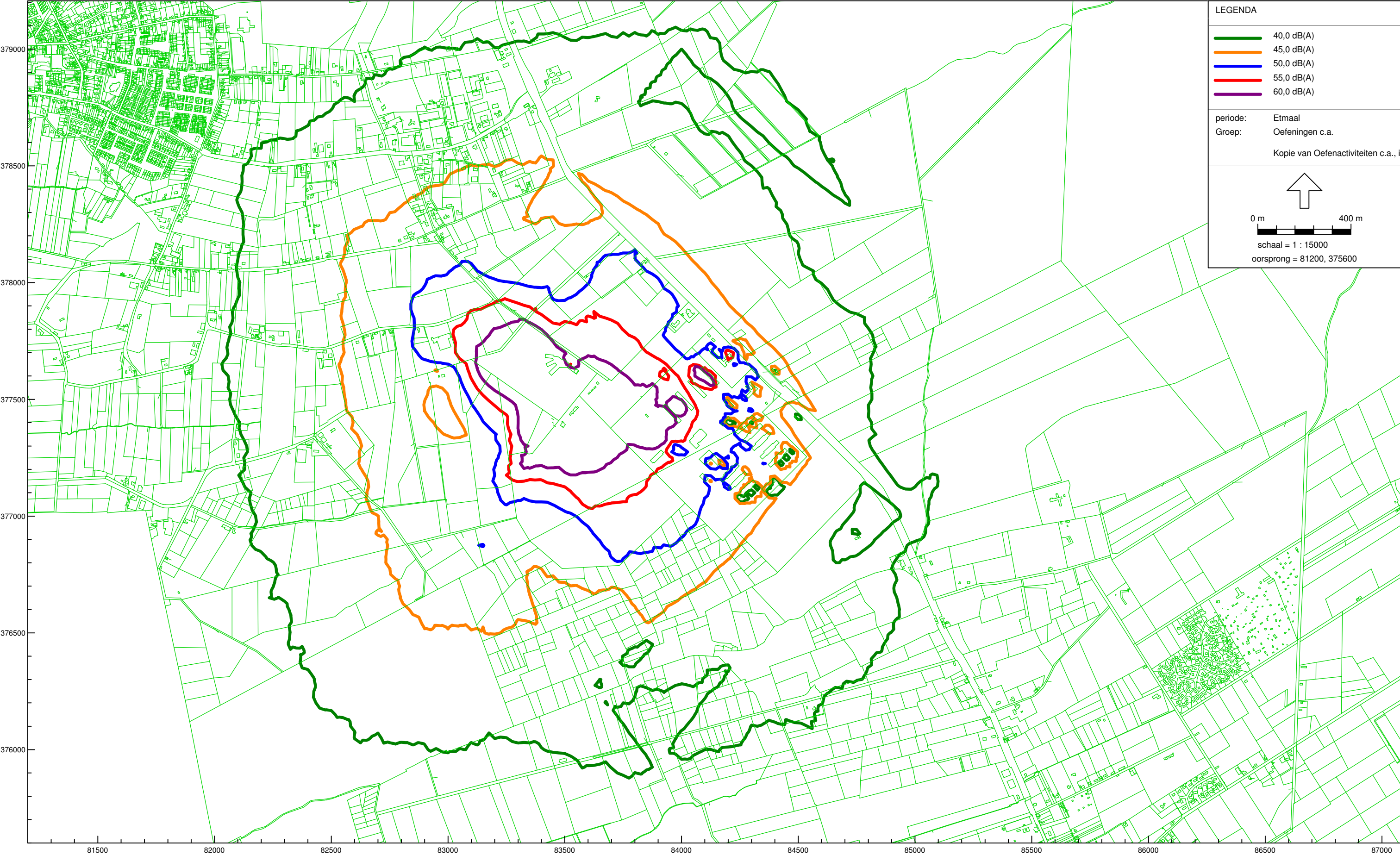
Figuur 3 LAr,LT-contouren
