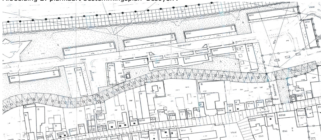
Afbeelding 2: plankaart bestemmingsplan 'Besoijen'.
