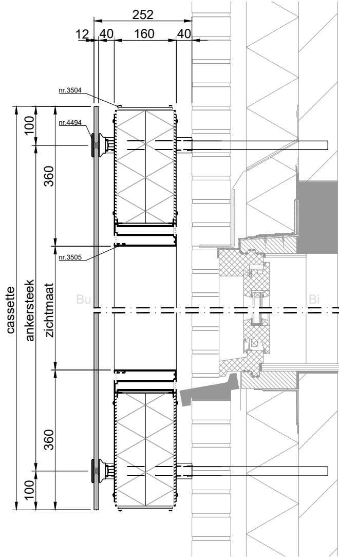
VERTICALE DOORSNEDE type SAG-10E-40
